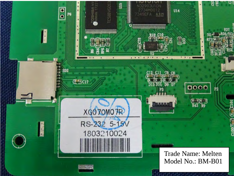
(40) EUT Photo
