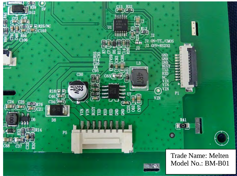
(44) EUT Photo
