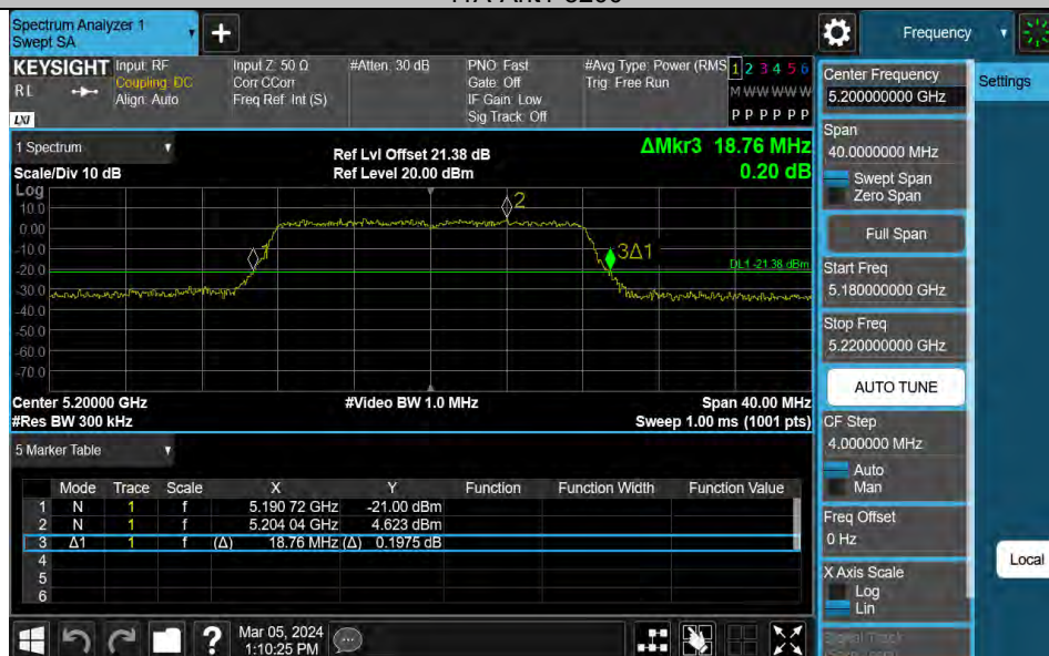
11A-Ant1-5200
