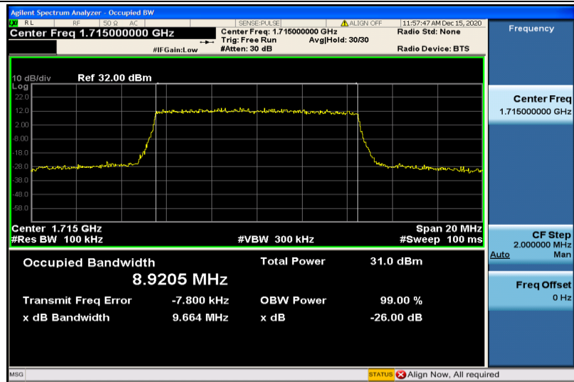
Band4-10MHz-QPSK-20000-50RB#0-8.9205
