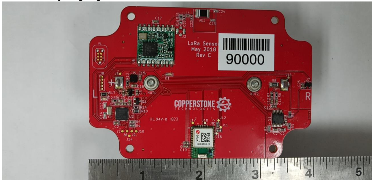
PCB assembly long edge
