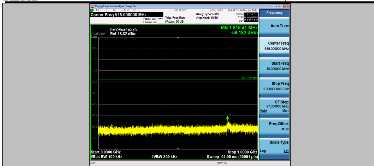
11G_Ant1_2462_30~1000
