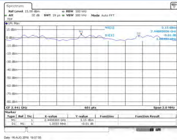
\Pi/4 -DQPSK
