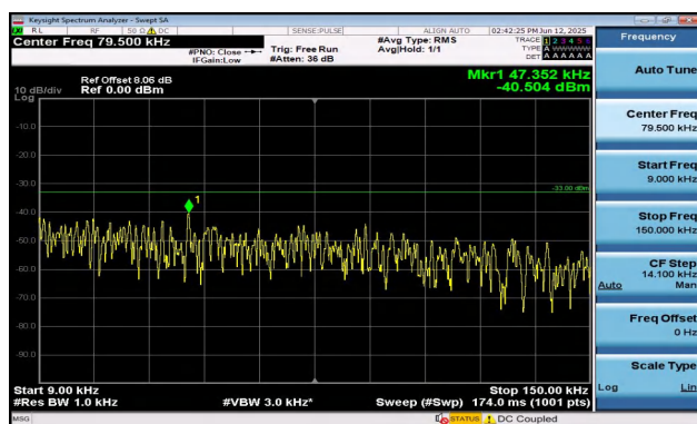
Band5-3MHz-QPSK-20635-15RB#0-0.009~0.15-PASS
