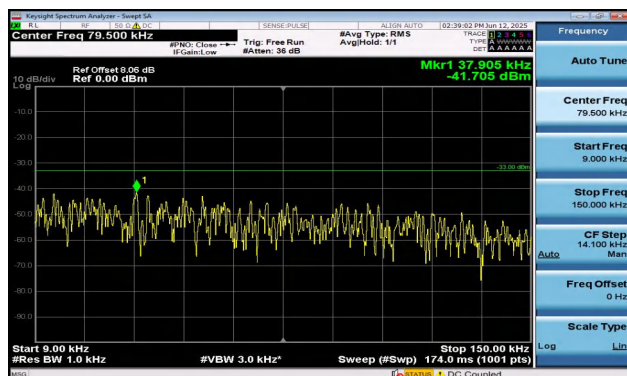
Band5-3MHz-QPSK-20635-1RB#0-0.009~0.15-PASS
