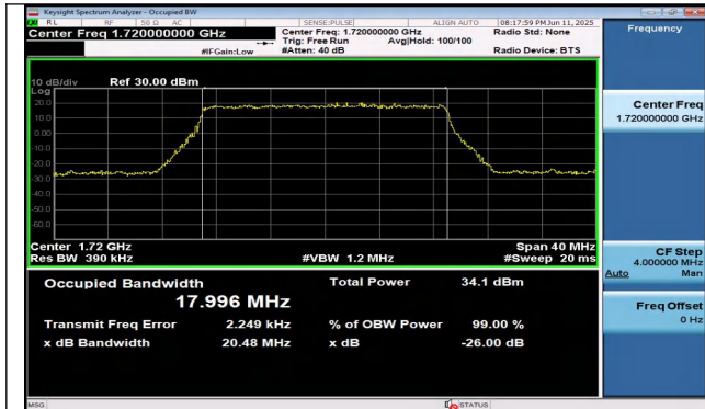
Band4-20MHz-QPSK-20050-100RB#0-PASS
