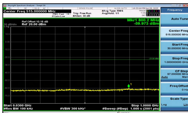
Band2-20MHz-QPSK-18700-1RB#0-30~1000-PASS
