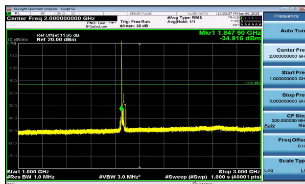
Band2-20MHz-QPSK-18700-1RB#0-1000~3000-PASS
