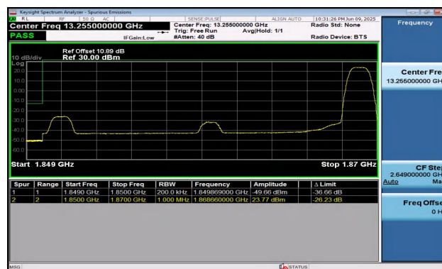
Band2-20MHz-QPSK-18700-1RB#99-PASS
