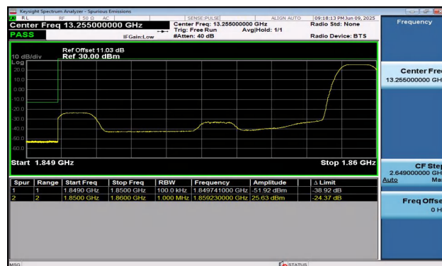
Band2-10MHz-QPSK-18650-1RB#49-PASS
