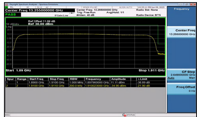
Band2-20MHz-QPSK-19100-100RB#0-PASS
