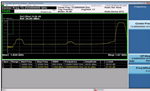
Band2-20MHz-16QAM-18700-1RB#99-PASS
