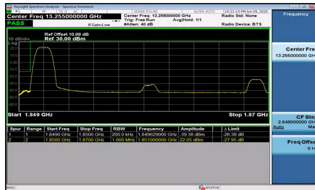
Band2-20MHz-16QAM-18700-1RB#0-PASS
