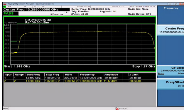
Band2-20MHz-QPSK-18700-100RB#0-PASS
