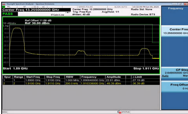
Band2-20MHz-16QAM-19100-1RB#0-PASS
