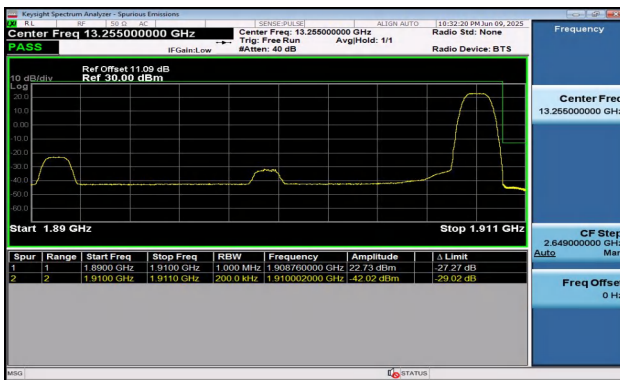
Band2-20MHz-QPSK-19100-1RB#99-PASS
