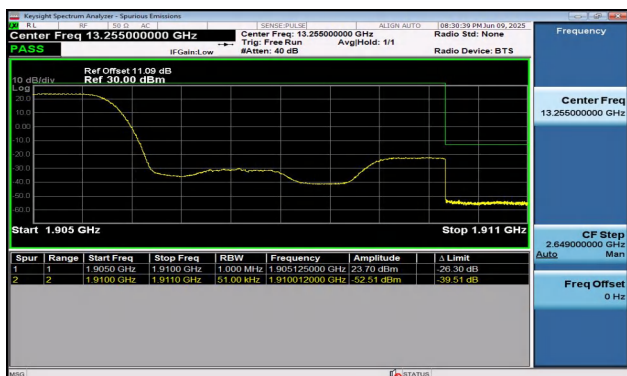
Band2-5MHz-QPSK-19175-1RB#0-PASS
