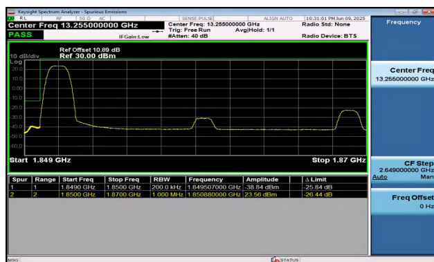
Band2-20MHz-QPSK-18700-1RB#0-PASS
