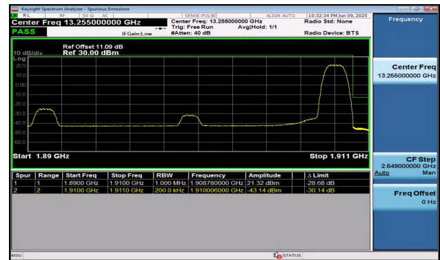
Band2-20MHz-16QAM-19100-1RB#99-PASS
