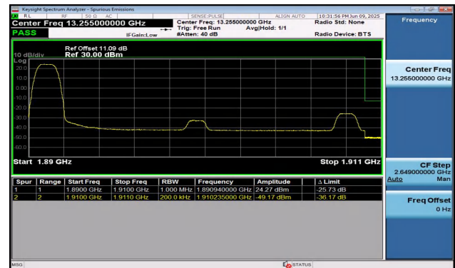
Band2-20MHz-QPSK-19100-1RB#0-PASS
