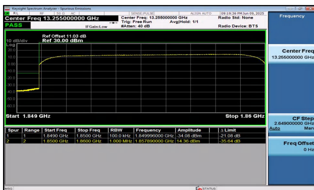
Band2-10MHz-QPSK-18650-50RB#0-PASS
