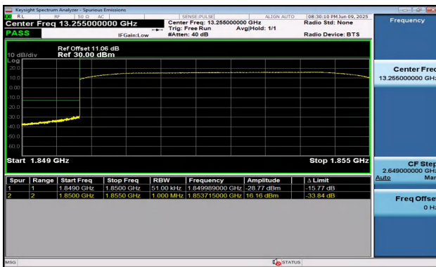
Band2-5MHz-QPSK-18625-25RB#0-PASS
