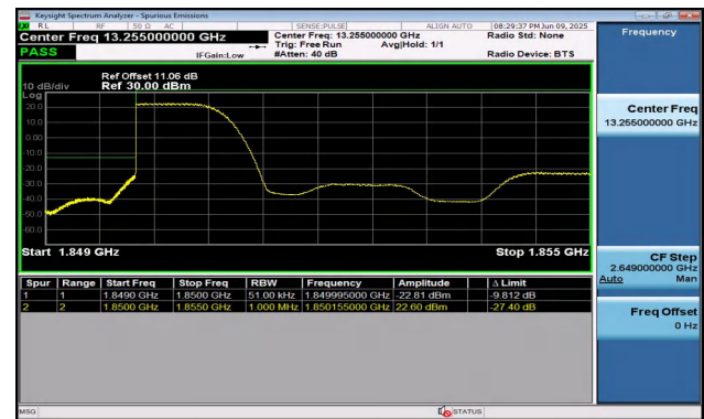
Band2-5MHz-16QAM-18625-1RB#0-PASS
