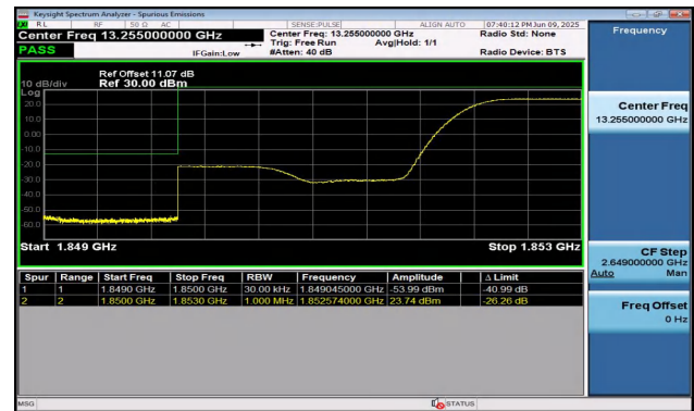
Band2-3MHz-QPSK-18615-1RB#14-PASS
