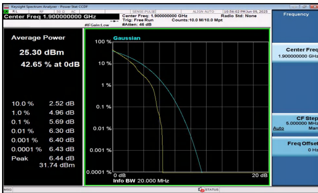
Band2-20MHz-QPSK-19100-1RB#0-PASS
