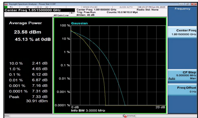
Band2-3MHz-QPSK-18615-15RB#0-PASS
