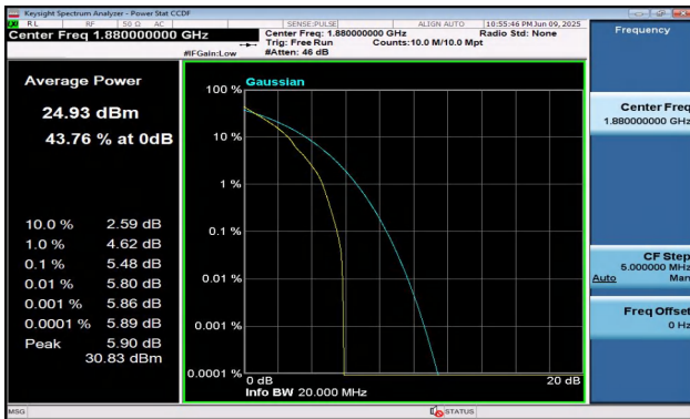
Band2-20MHz-QPSK-18900-1RB#0-PASS
