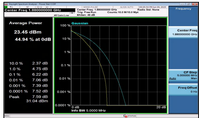
Band2-5MHz-QPSK-18900-25RB#0-PASS
