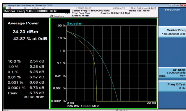
Band2-10MHz-QPSK-18650-1RB#0-PASS
