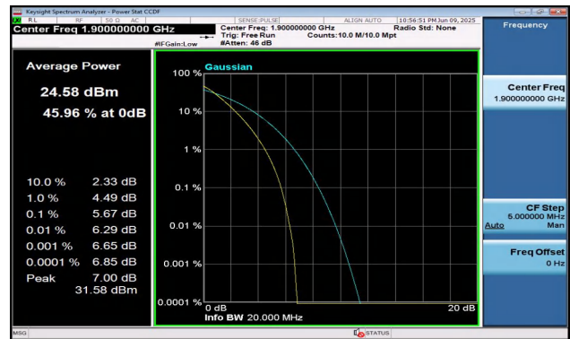
Band2-20MHz-QPSK-19100-100RB#0-PASS
