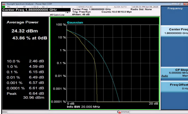
Band2-20MHz-QPSK-18700-1RB#0-PASS
