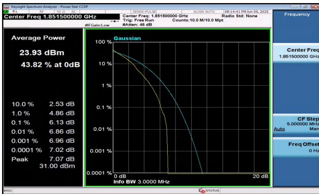
Band2-3MHz-QPSK-18615-1RB#0-PASS
