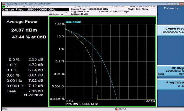
Band2-3MHz-QPSK-18900-1RB#0-PASS
