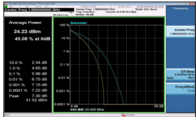
Band2-20MHz-QPSK-18900-100RB#0-PASS
