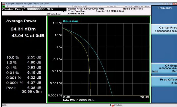
Band2-5MHz-QPSK-18900-1RB#0-PASS
