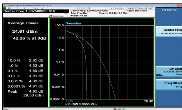
Band2-5MHz-QPSK-19175-1RB#0-PASS
