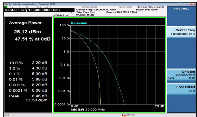
Band2-20MHz-QPSK-18700-100RB#0-PASS
