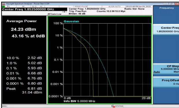
Band2-5MHz-QPSK-18625-1RB#0-PASS
