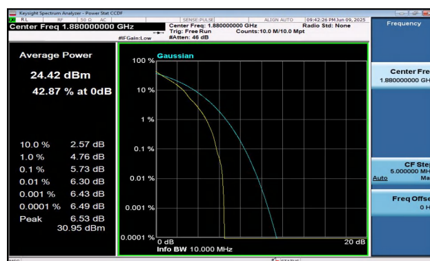
Band2-10MHz-QPSK-18900-1RB#0-PASS
