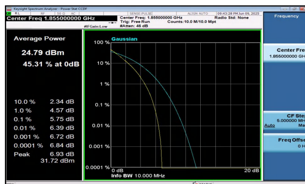
Band2-10MHz-QPSK-18650-50RB#0-PASS
