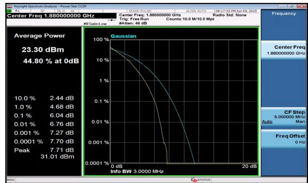
Band2-3MHz-QPSK-18900-15RB#0-PASS
