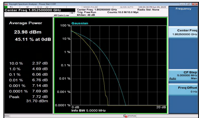
Band2-5MHz-QPSK-18625-25RB#0-PASS
