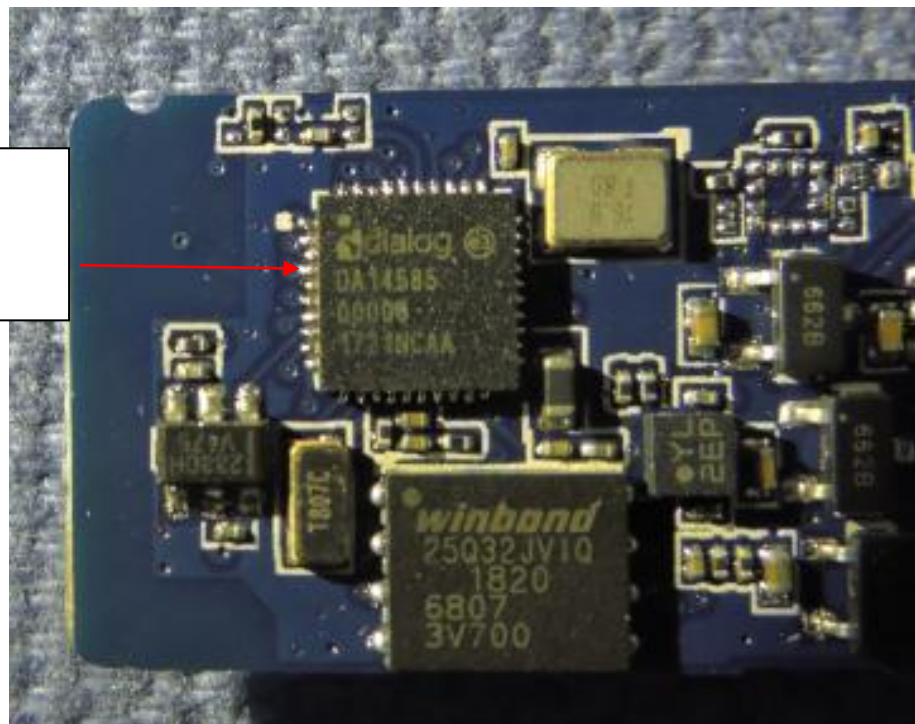
BLE Chip
