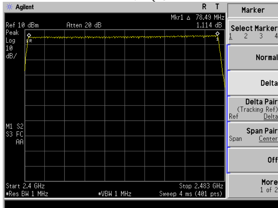
Pi/4 DQPSK
