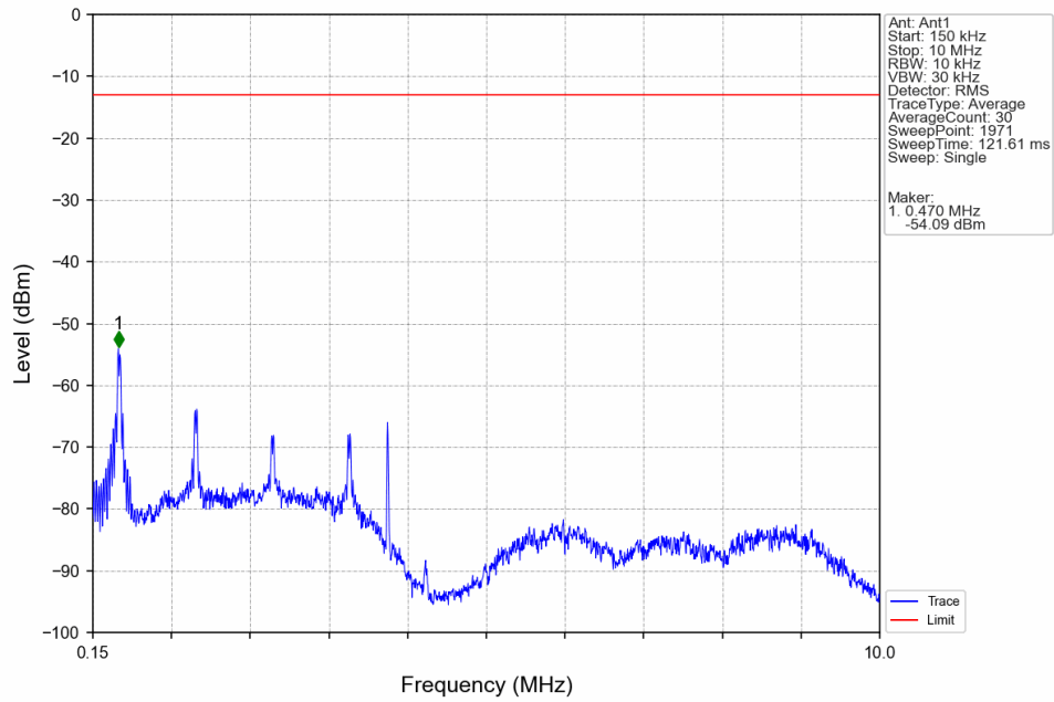
Band4_HSUPA_LCH_1712.4MHz_Subtest 1_NTNV
