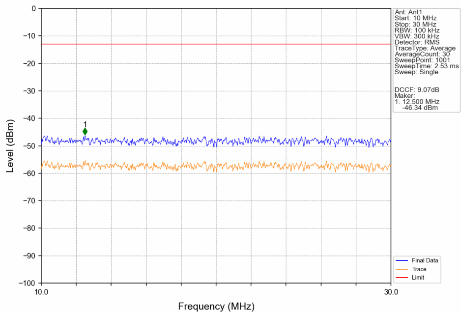
GSM850_GSM_LCH_824.2MHz_GSM_NTNV
