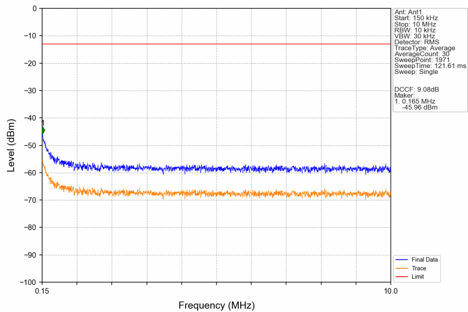
GSM850_GSM_HCH_848.8MHz_GSM_NTNV
