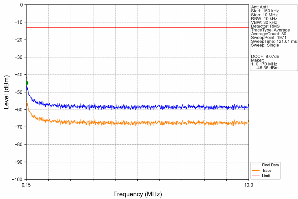
GSM850_GSM_LCH_824.2MHz_GSM_NTNV
