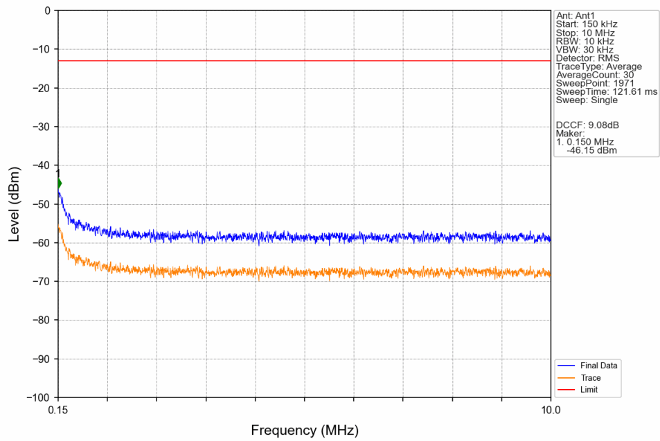
GSM850_GSM_MCH_836.6MHz_GSM_NTNV
