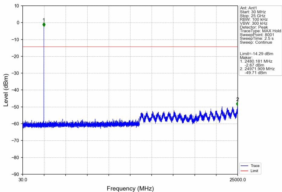
Pi/4DQPSK 2DH5 HCH 2480MHz Ant1 NTV
