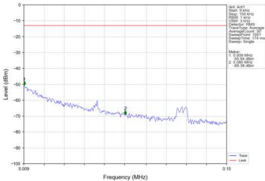
Band4 HSUPA LCH 1712.4MHz Subtest 1 NTV
