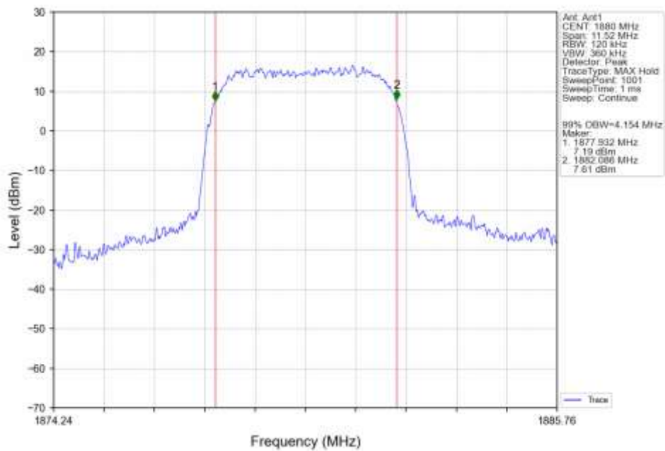
Band2 HSUPA MCH 1880MHz Subtest 1 NTV
