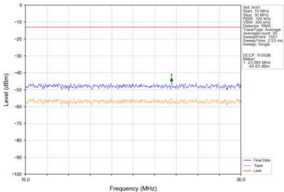
GSM850_GPRS_HCH_848.8MHz_1_TX_Slot_NTNV
