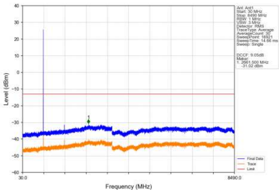
GSM850_GPRS_HCH_848.8MHz_1_TX_Slot_NTNV
