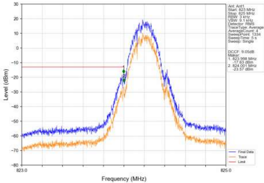
GSM850_GSM_LCH_824.2MHz_GSM_NTNV
