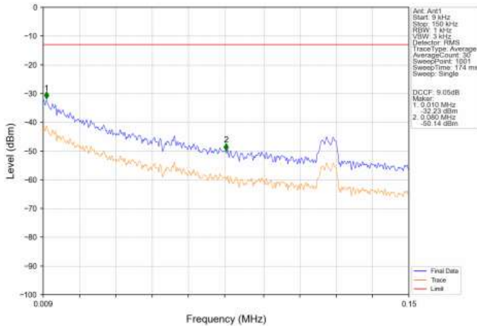
GSM850_GSM_LCH_824.2MHz_GSM_NTNV
