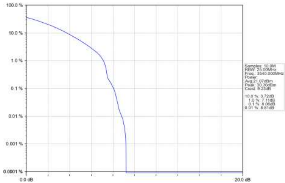
n78e 30kHz SISO NTN 20MHz CP-OFDM 256 QAM 3540MHz Outer Full Ant1
