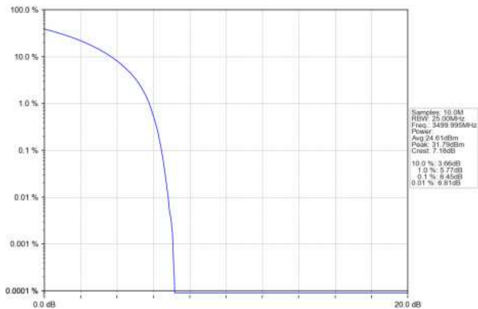
n78e 15kHz SISO NTV 20MHz CP-OFDM QPSK 3499.995MHz Outer Full Ant1
