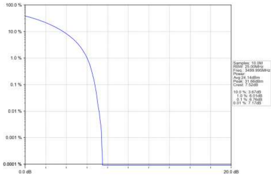
n78e 15kHz SISO NTN 20MHz CP-OFDM 64 QAM 3499.995MHz Outer Full Ant1
