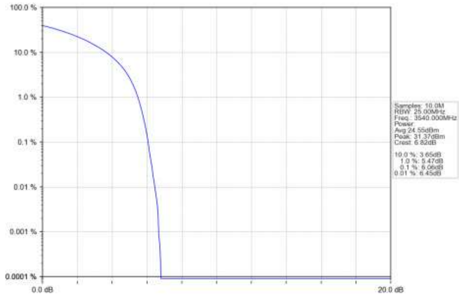
n78e 15kHz SISO NTN 20MHz CP-OFDM 64 QAM 3540MHz Outer Full Ant1
