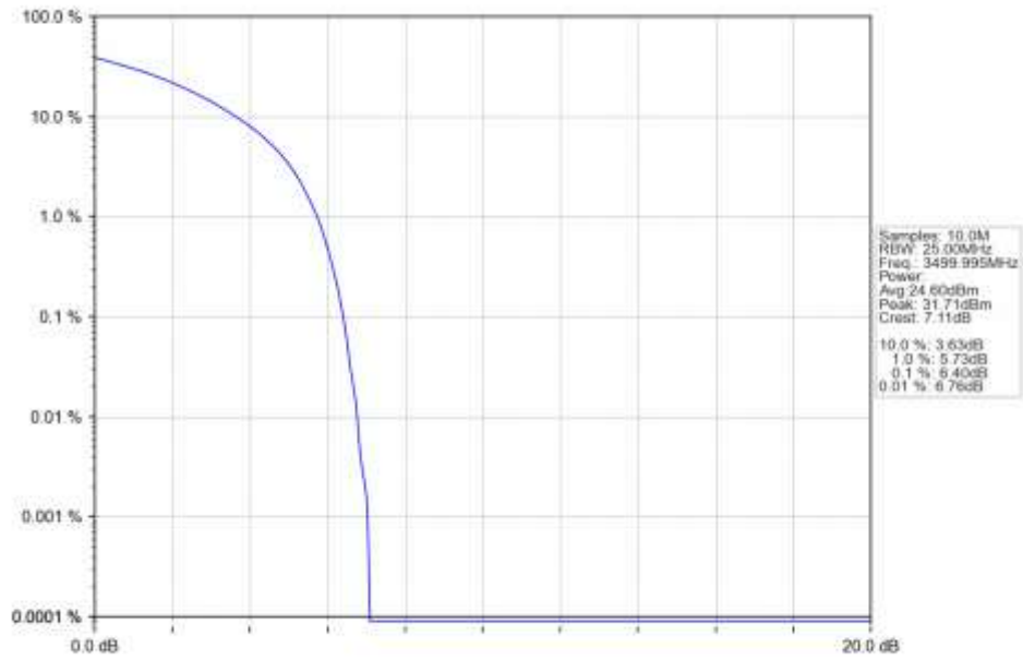
n78e 15kHz SISO NTN 20MHz CP-OFDM 16 QAM 3499.995MHz Outer Full Ant1
