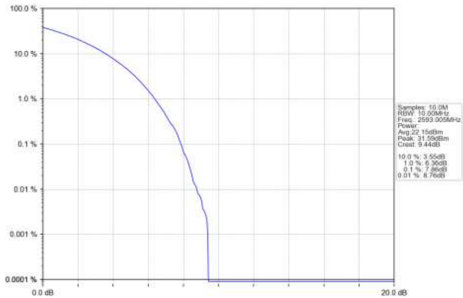
n41 15kHz SISO NTN 10MHz CP-OFDM QPSK 2593.005MHz Outer Full Ant1
