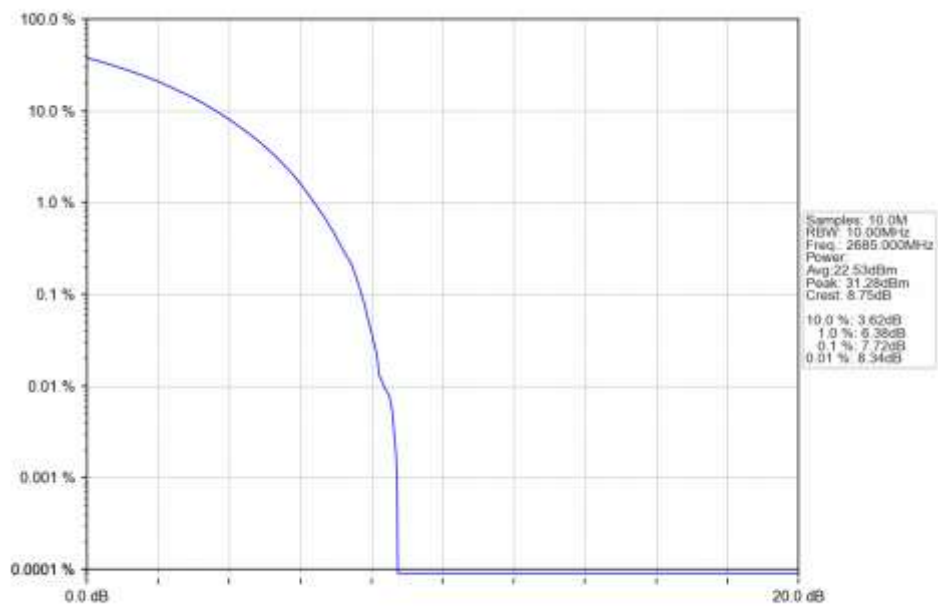
n41 15kHz SISO NTN 10MHz CP-OFDM QPSK 2685MHz Outer Full Ant1
