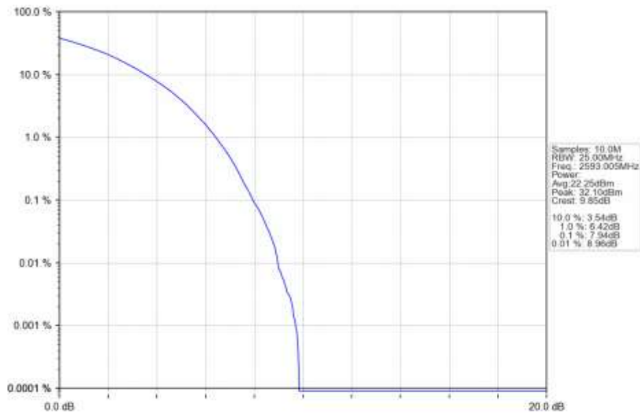
n41 15kHz SISO NTN 20MHz CP-OFDM QPSK 2593.005MHz Outer Full Ant1
