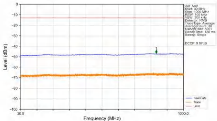
n78a 30kHz SISO NTN 60MHz CP-OFDM QPSK 3750MHz Edge 1RB Left Ant1
