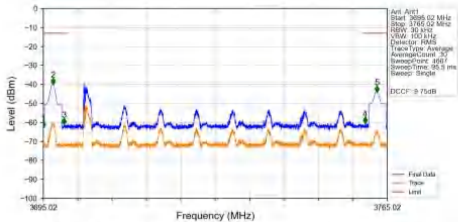
n78a 30kHz SISO NTN 60MHz CP-OFDM QPSK 3730.02MHz Inner 1RB Left Ant1
