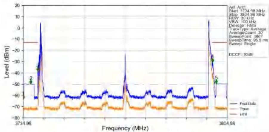
n78a 30kHz SISO NTN 60MHz CP-OFDM QPSK 3769.98MHz Inner_1RB_Right_Ant1
