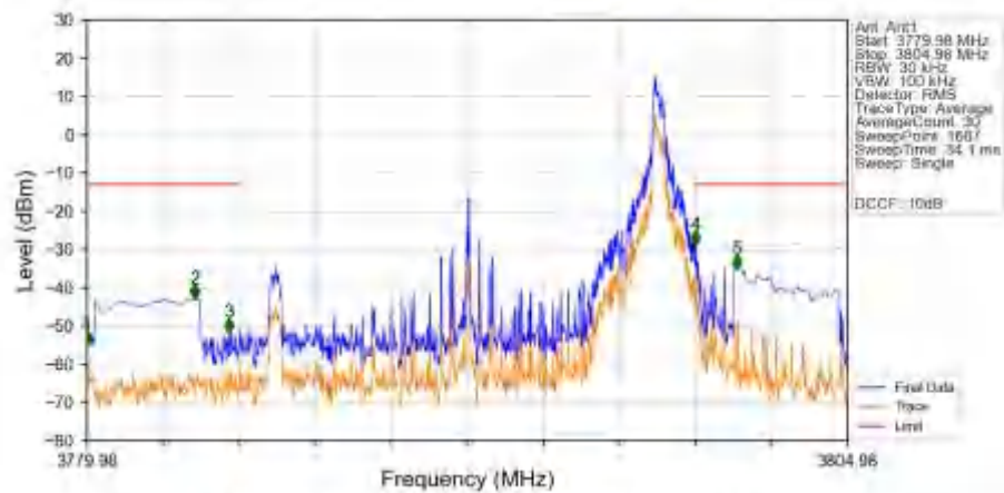
n78a 30kHz SISO NTN 15MHz CP-OFDM QPSK 3792.48MHz Inner_1RB_Right_Ant1
