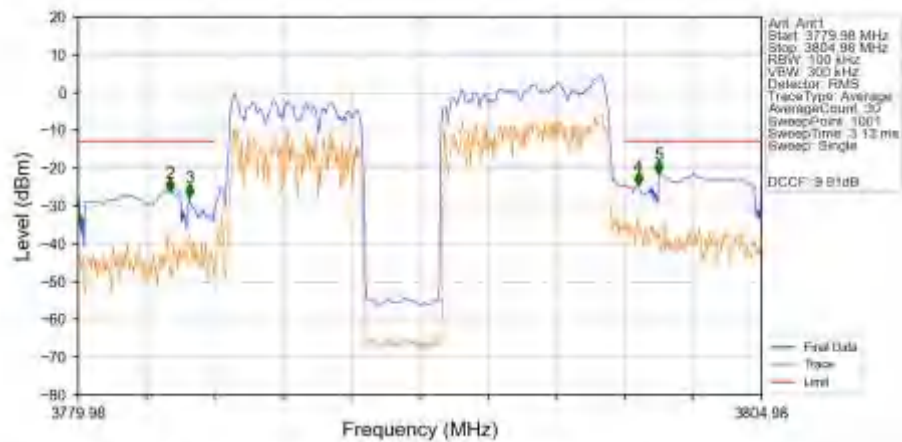
n78a 30kHz SISO NTN 15MHz CP-OFDM QPSK 3792.48MHz Outer_Full_Ant1
