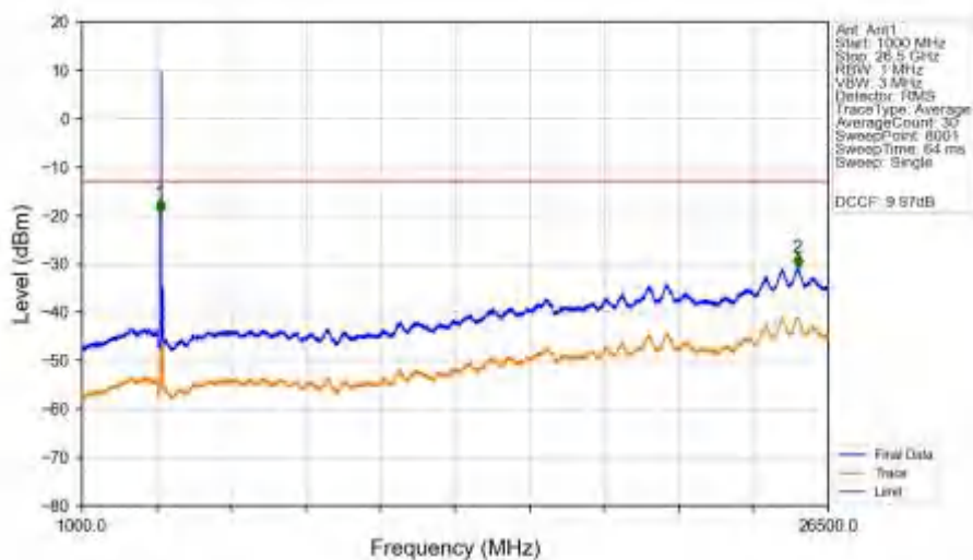
n78a 30kHz SISO NTN 80MHz CP-OFDM QPSK 3750MHz Edge 1RB Left Ant1
