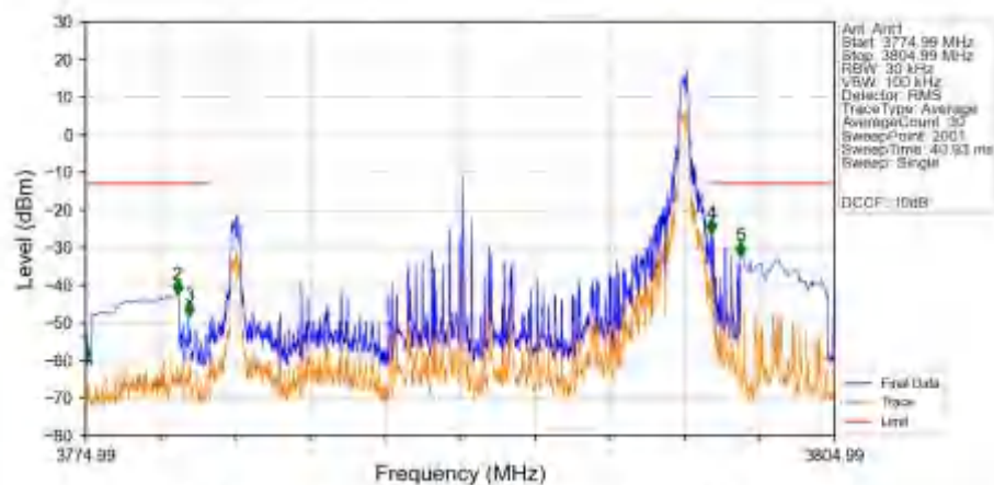
n78a 30kHz SISO NTN 20MHz DFT-s-OFDM QPSK 3789.99MHz Edge 1RB Right Ant1
