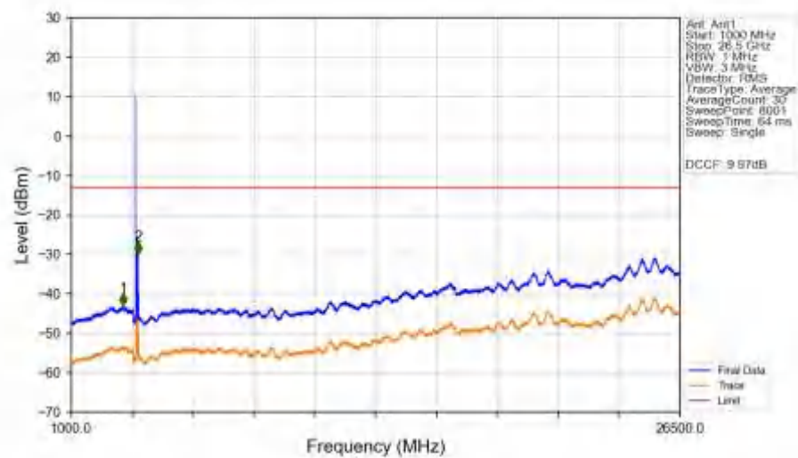
n78a 30kHz SISO NTN 50MHz DFT-s-OFDM QPSK 3725.01MHz Edge 1RB Left Ant1
