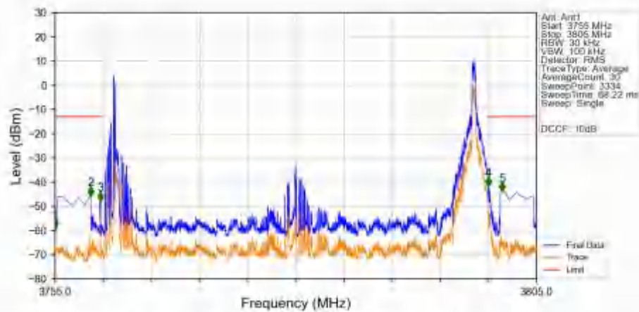
n78a 30kHz SISO NTN 40MHz DFT-s-OFDM QPSK 3780MHz Inner 1RB Right Ant1
