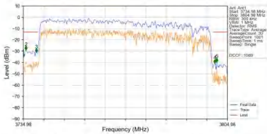
n78a 30kHz SISO NTN 60MHz CP-OFDM QPSK 3769.98MHz Outer_Full_Ant1
