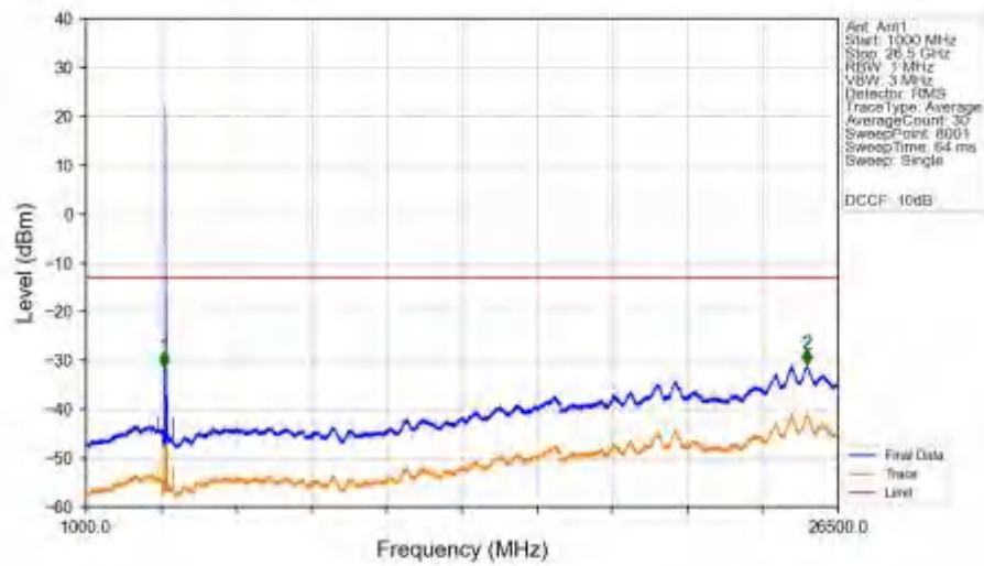
n78a 30kHz SISO NTN 20MHz DFT-s-OFDM QPSK 3710.01MHz Edge 1RB Left Ant1
