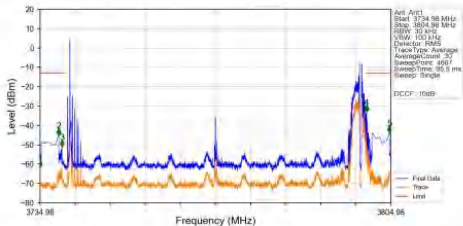
n78a 30kHz SISO NTN 60MHz CP-OFDM QPSK 3769.98MHz Edge 1RB Right Ant1
