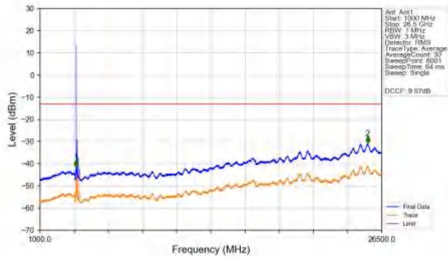
n78a 30kHz SISO NTN 80MHz DFT-s-OFDM QPSK 3740.01MHz Edge 1RB Left Ant1
