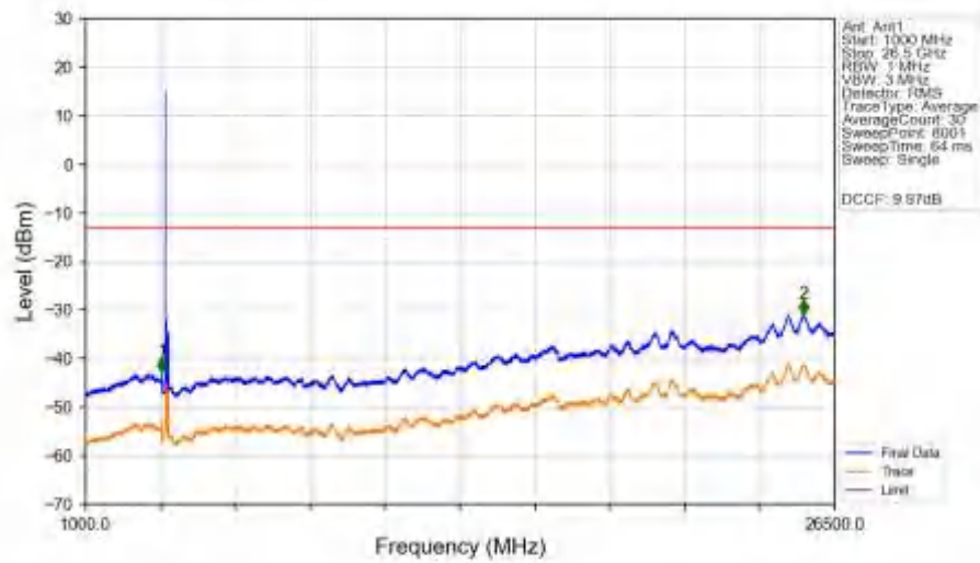
n78a 30kHz SISO NTN 60MHz CP-OFDM QPSK 3750MHz Edge 1RB Left Ant1
