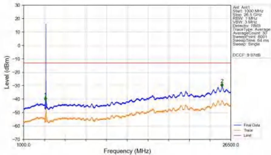
n78a 30kHz SISO NTN 30MHz DFT-s-OFDM QPSK 3750MHz Edge 1RB Left Ant1
