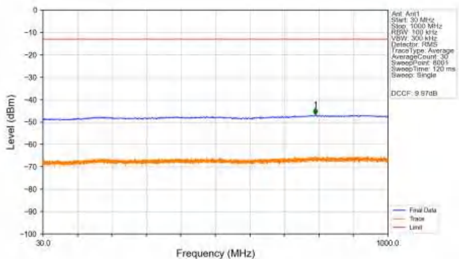
n78a 30kHz SISO NTN 60MHz DFT-s-OFDM QPSK 3750MHz Edge 1RB Left Ant1
