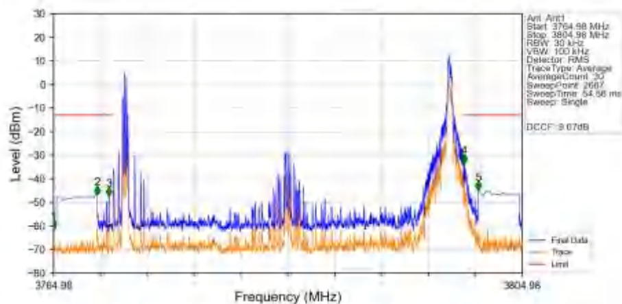
n78a 30kHz SISO NTN 30MHz DFT-s-OFDM QPSK 3784.98MHz Edge 1RB Right Ant1
