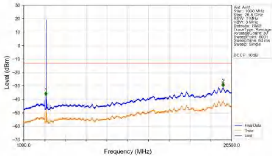
n78a 30kHz SISO NTN 20MHz DFT-s-OFDM QPSK 3750MHz Edge 1RB Left Ant1
