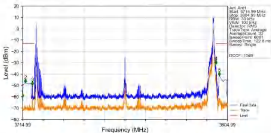
n78a 30kHz SISO NTN 80MHz CP-OFDM QPSK 3759.99MHz Edge 1RB Right Ant1
