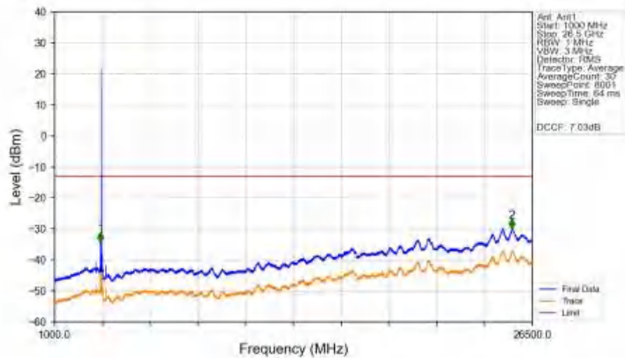
n77d_15kHz_SISO_NTNV_20MHz_CP-OFDM_QPSK_3499.995MHz_Edge_1RB_Left_Ant1
