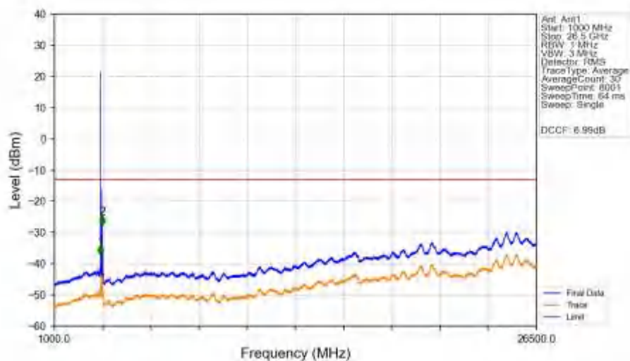
n77d 15kHz SISO NTN 40MHz DFT-s-OFDM QPSK 3470.01MHz Edge 1RB Left Ant1
