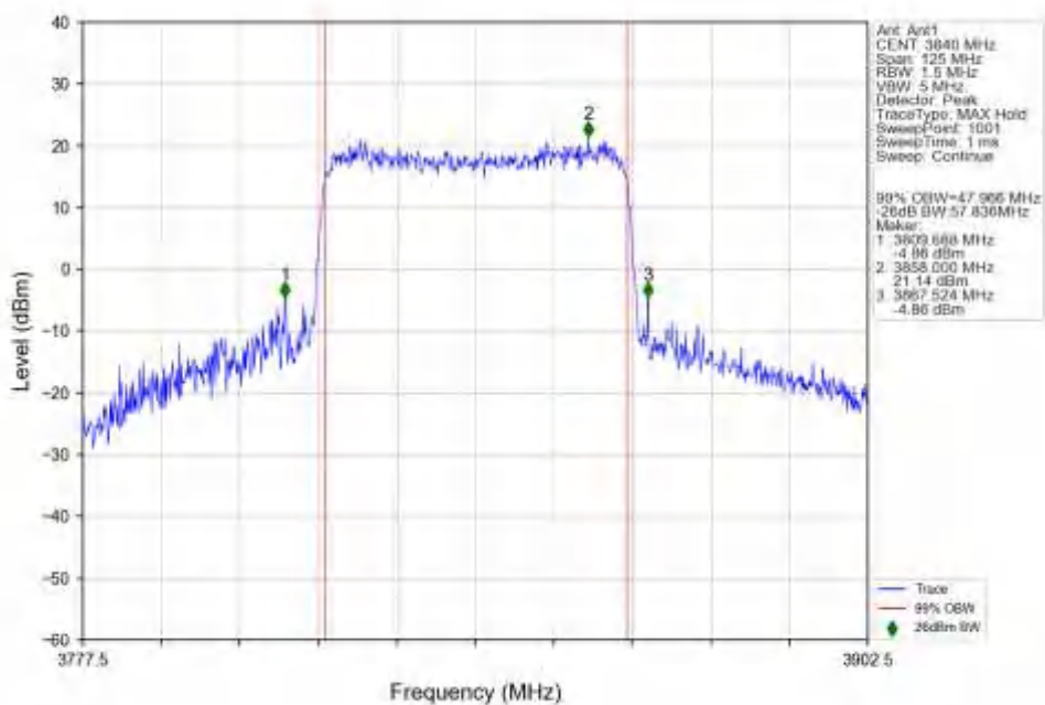
n77a 30kHz SISO_NTNV_50MHz CP-OFDM QPSK 3840MHz_Outer_Full_Ant1
