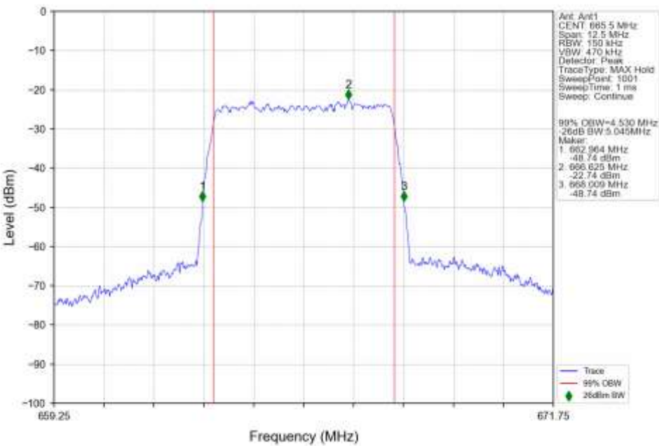
n71_15kHz_SISO_NTNV_5MHz_CP-OFDM_256_QAM_665.5MHz_Outer_Full_Ant1
