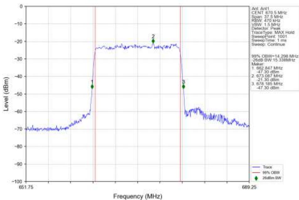
n71_15kHz_SISO_NTNV_15MHz_CP-OFDM_256_QAM_670.5MHz_Outer_Full_Ant1
