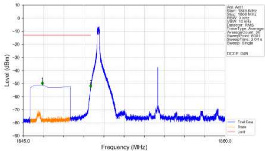
n2_15kHz_SISO_NTNV_10MHz_DFT-s-OFDM_QPSK_1855MHz_Inner_1RB_Left_Ant1
