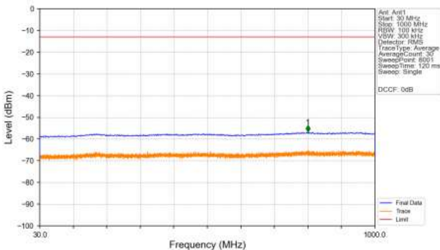
n2_15kHz_SISO_NTNV_10MHz_CP-OFDM_QPSK_1880MHz_Edge_1RB_Left_Ant1
