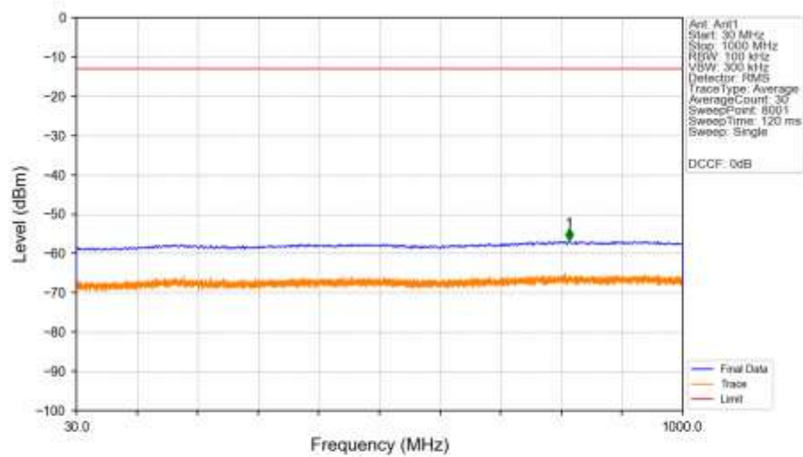
n2_30kHz_SISO_NTNV_20MHz_CP-OFDM_QPSK_1860MHz_Edge_1RB_Left_Ant1
