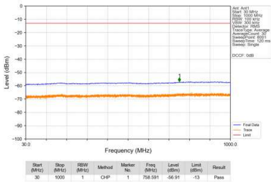
n2_30kHz_SISO_NTNV_10MHz_CP-OFDM_QPSK_1855MHz_Edge_1RB_Left_Ant1
