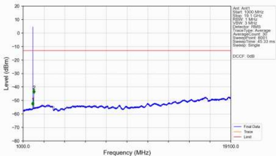
n2_30kHz_SISO_NTNV_10MHz_DFT-s-OFDM_QPSK_1855MHz_Edge_1RB_Left_Ant1
