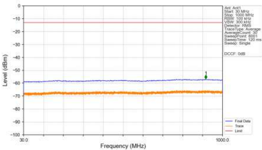
n2_30kHz_SISO_NTNV_10MHz_CP-OFDM_QPSK_1880MHz_Edge_1RB_Left_Ant1
