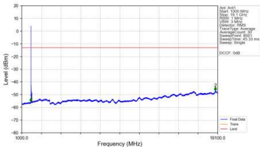
n2_30kHz_SISO_NTNV_20MHz_CP-OFDM_QPSK_1860MHz_Edge_1RB_Left_Ant1
