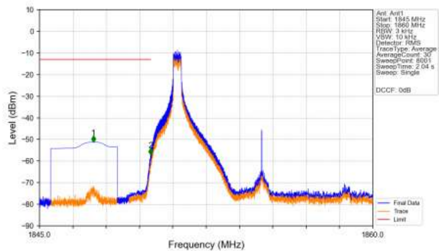
n2_30kHz_SISO_NTNV_10MHz_CP-OFDM_QPSK_1855MHz_Inner_1RB_Left_Ant1
