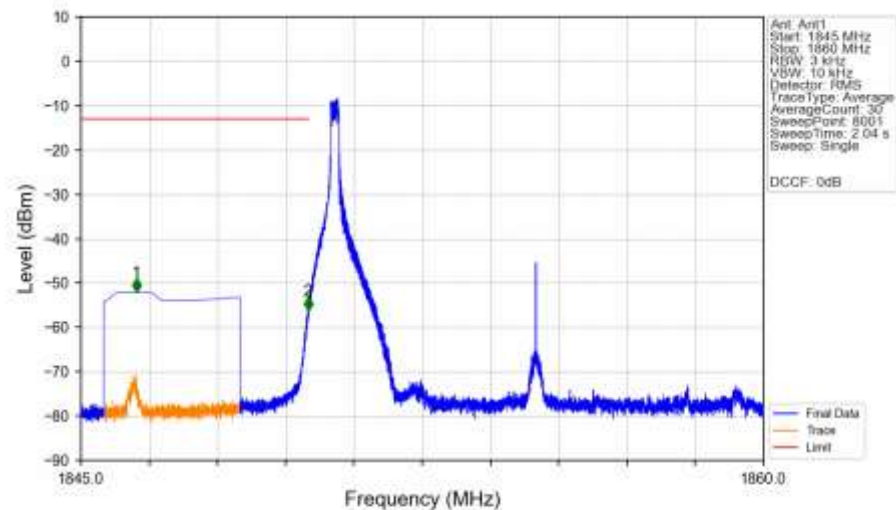
n2_15kHz_SISO_NTNV_10MHz_CP-OFDM_QPSK_1855MHz_Inner_1RB_Left_Ant1
