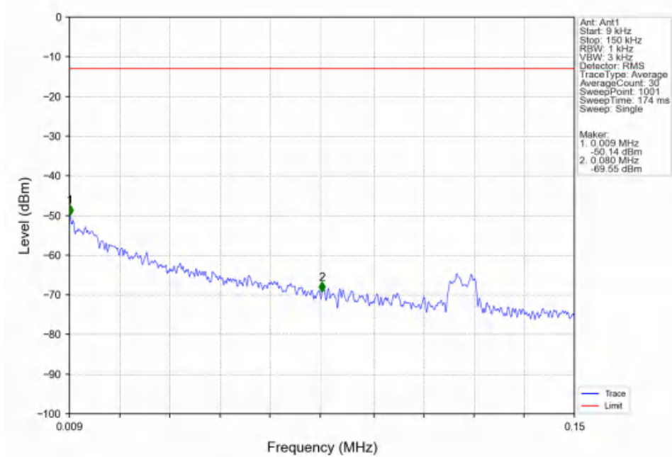
Band25_20MHz_QPSK_HCH_1905MHz_RB_1_0_NTNV
