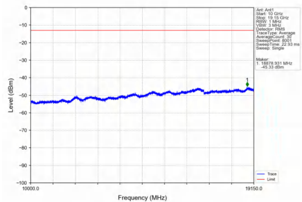
Band25_10MHz_QPSK_HCH_1910MHz_RB_1_49_NTNV
