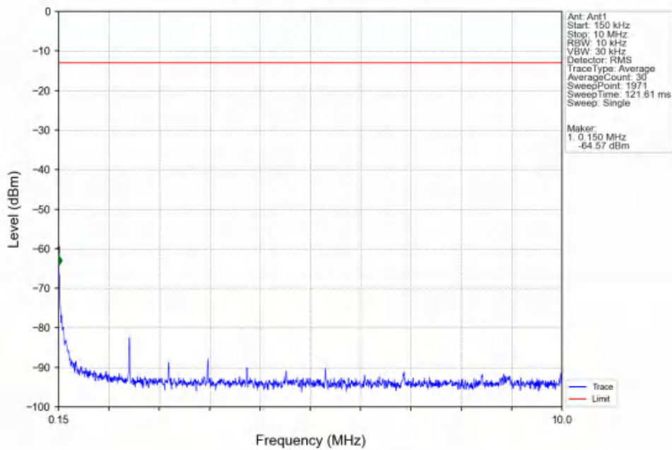
Band25 20MHz_QPSK_LCH_1860MHz_RB_1_0_NTNV
