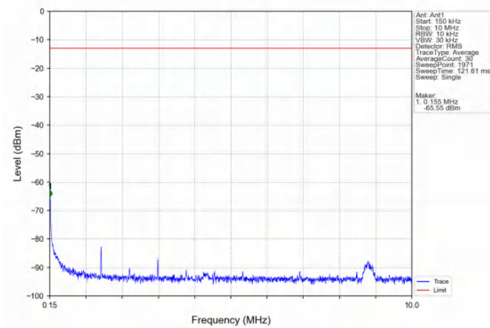
Band25_10MHz_QPSK_HCH_1910MHz_RB_1_0_NTNV
