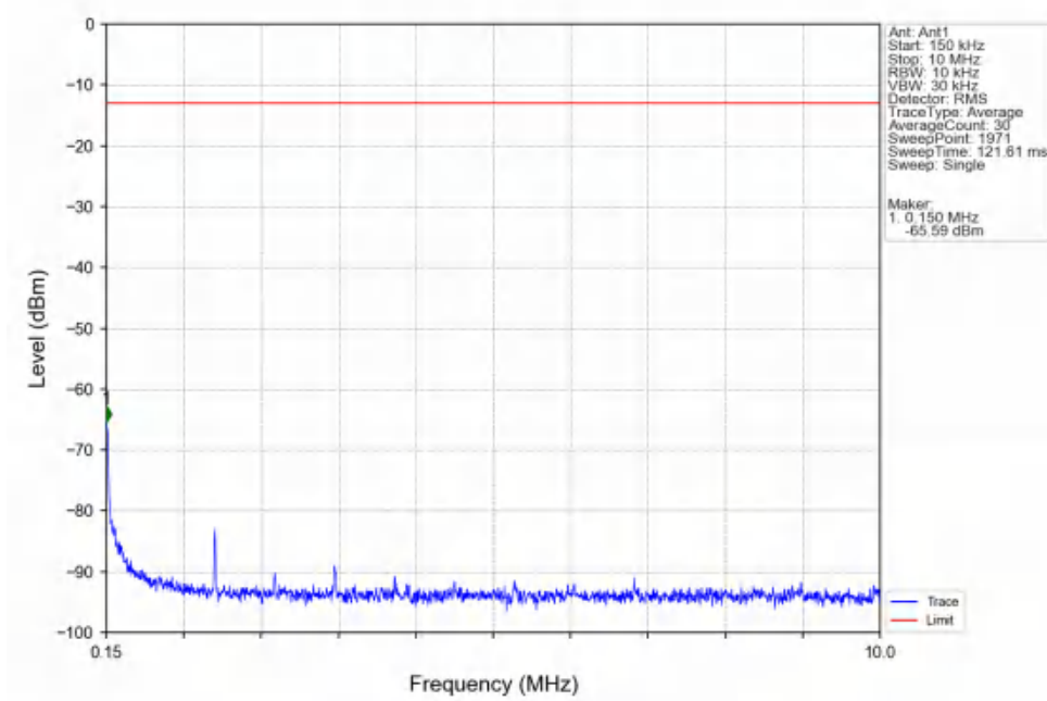
Band25_20MHz_QPSK_HCH_1905MHz_RB_1_0_NTNV
