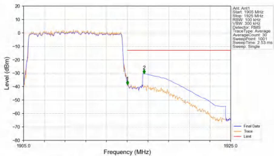
Band25_10MHz_QPSK_HCH_1910MHz_RB_50_0_NTNV
