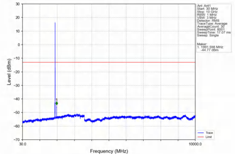
Band25_10MHz_QPSK_HCH_1910MHz_RB_1_0_NTNV
