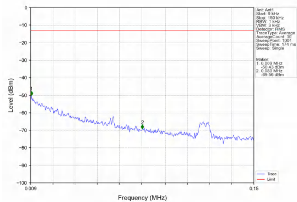
Band25_10MHz_QPSK_HCH_1910MHz_RB_1_0_NTNV
