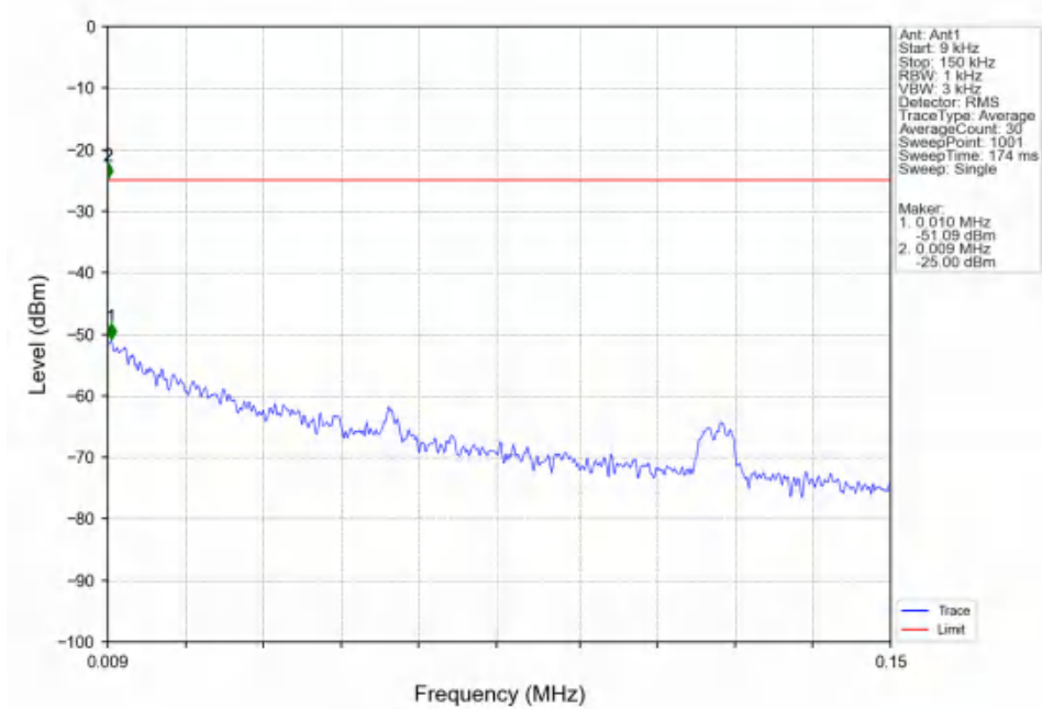
Band7_20MHz_16QAM_HCH_2560MHz_RB_1_0_NTNV
