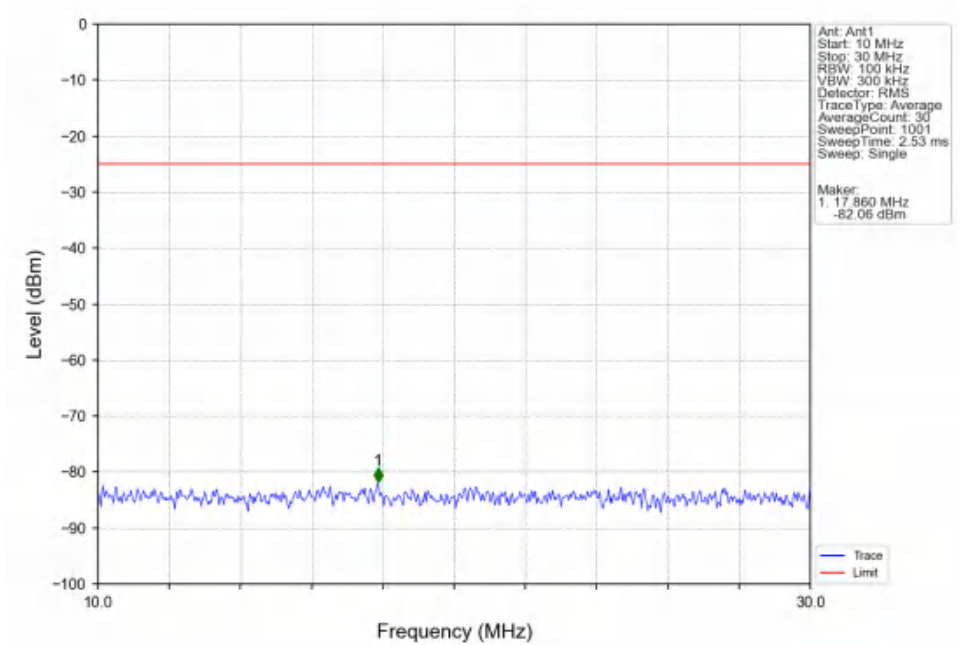
Band7_20MHz_QPSK_HCH_2560MHz_RB_1_0_NTNV
