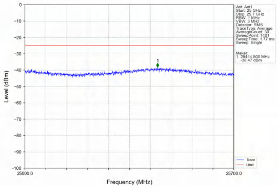
Band7_20MHz_QPSK_HCH_2560MHz_RB_1_0_NTNV
