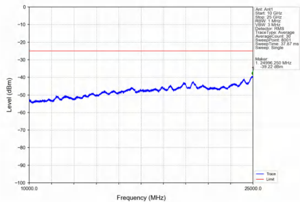
Band7_20MHz_16QAM_LCH_2510MHz_RB_1_0_NTNV
