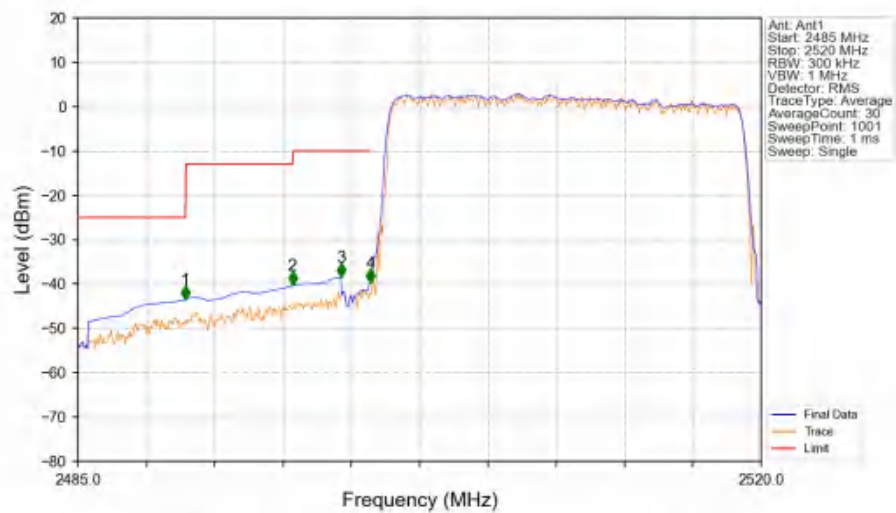
Band7_20MHz_QPSK_LCH_2510MHz_RB_100_0_NTNV
