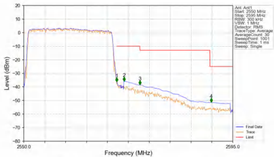
Band7_20MHz_16QAM_HCH_2560MHz_RB_100_0_NTNV
