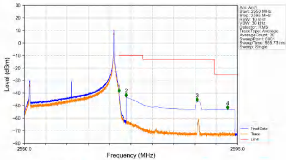
Band7_20MHz_16QAM_HCH_2560MHz_RB_1_99_NTNV
