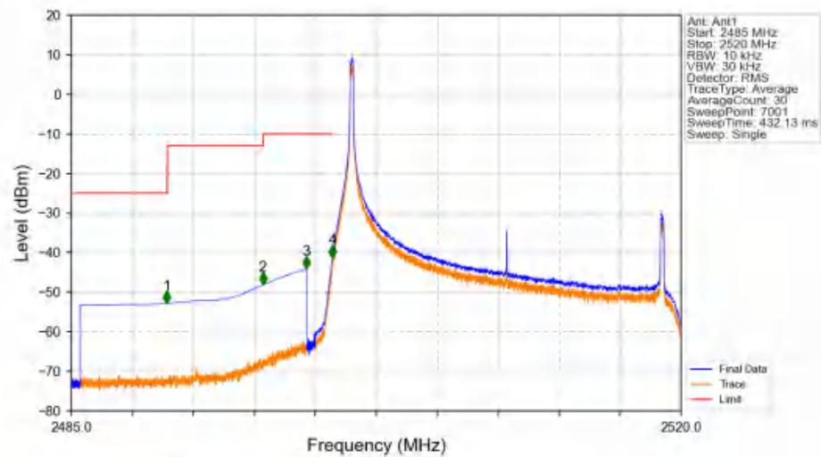
Band7_20MHz_16QAM_LCH_2510MHz_RB_1_0_NTNV
