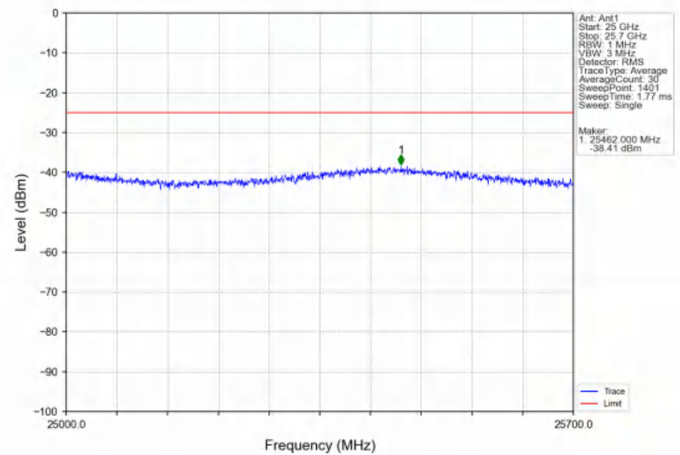
Band7_20MHz_QPSK_MCH_2535MHz_RB_1_0_NTNV
