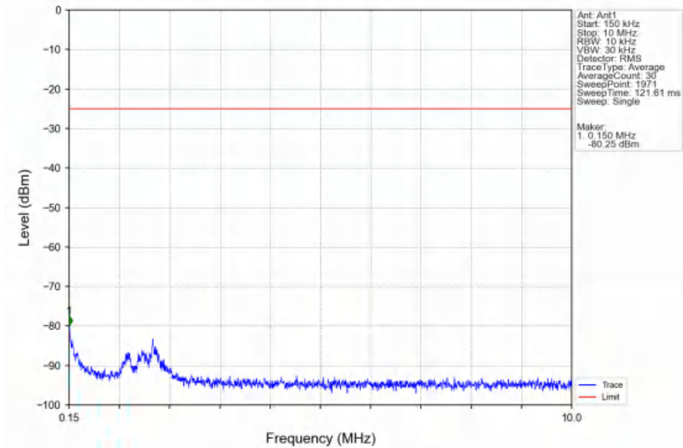
Band7_20MHz_QPSK_LCH_2510MHz_RB_1_0_NTNV
