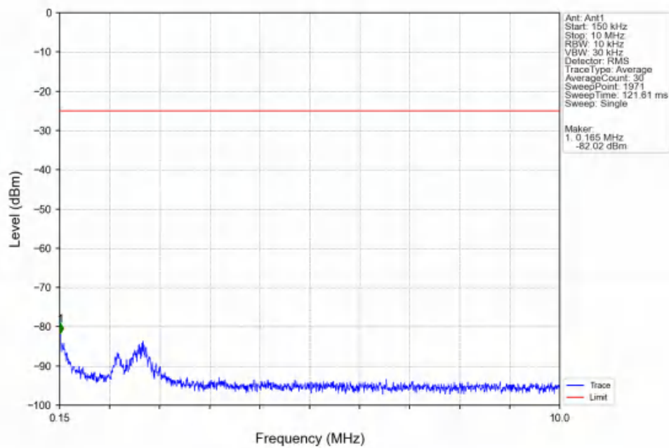
Band7_20MHz_16QAM_MCH_2535MHz_RB_1_0_NTNV
