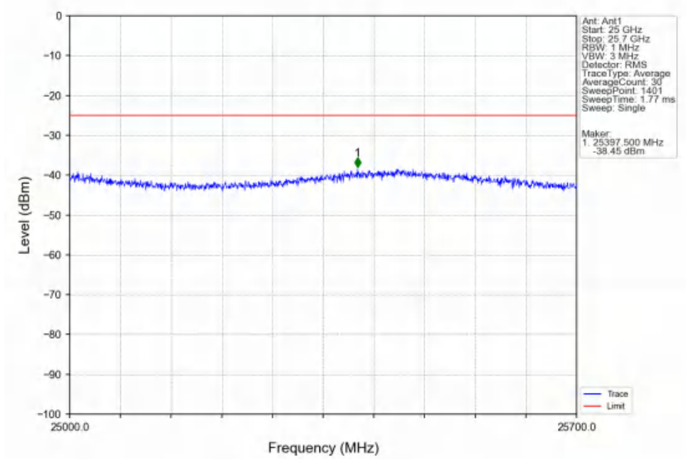
Band7_20MHz_16QAM_HCH_2560MHz_RB_1_0_NTNV
