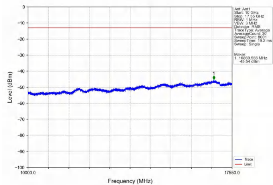
Band4_15MHz_QPSK_HCH_1747.5MHz_RB_1_74_NTNV
