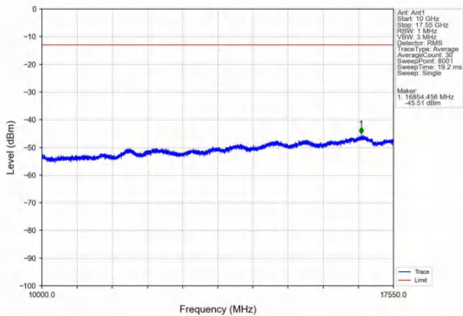
Band4_10MHz_QPSK_HCH_1750MHz_RB_1_49_NTNV
