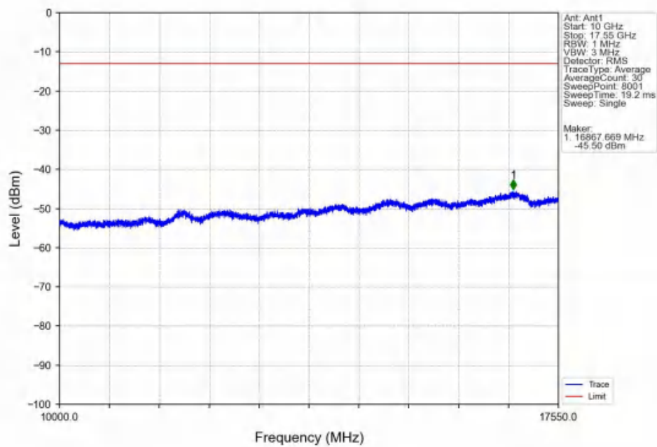
Band4_20MHz_QPSK_HCH_1745MHz_RB_1_99_NTNV
