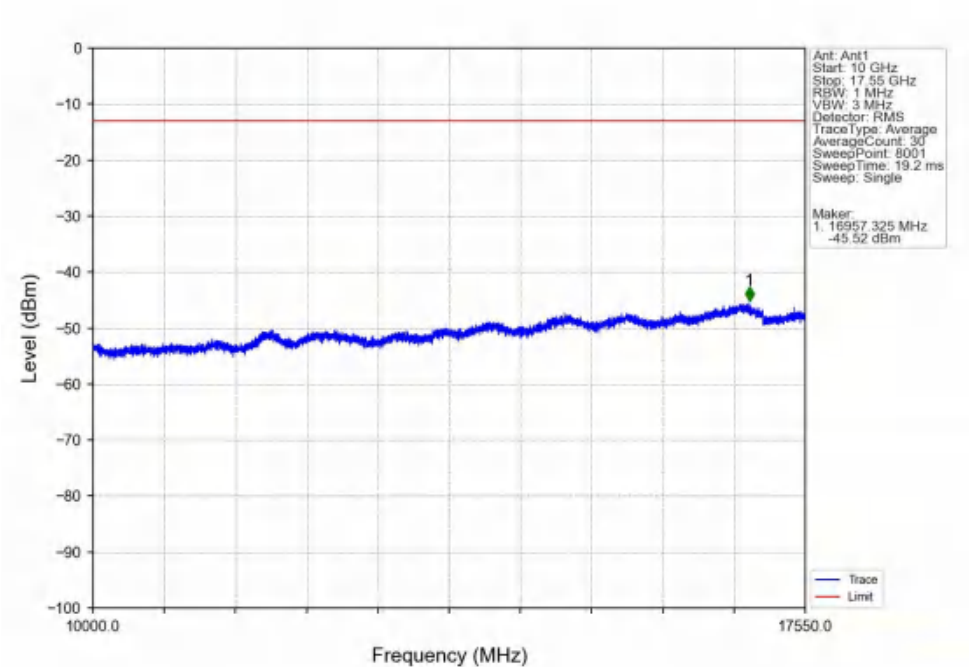
Band4_20MHz_QPSK_MCH_1732.5MHz_RB_1_0_NTNV
