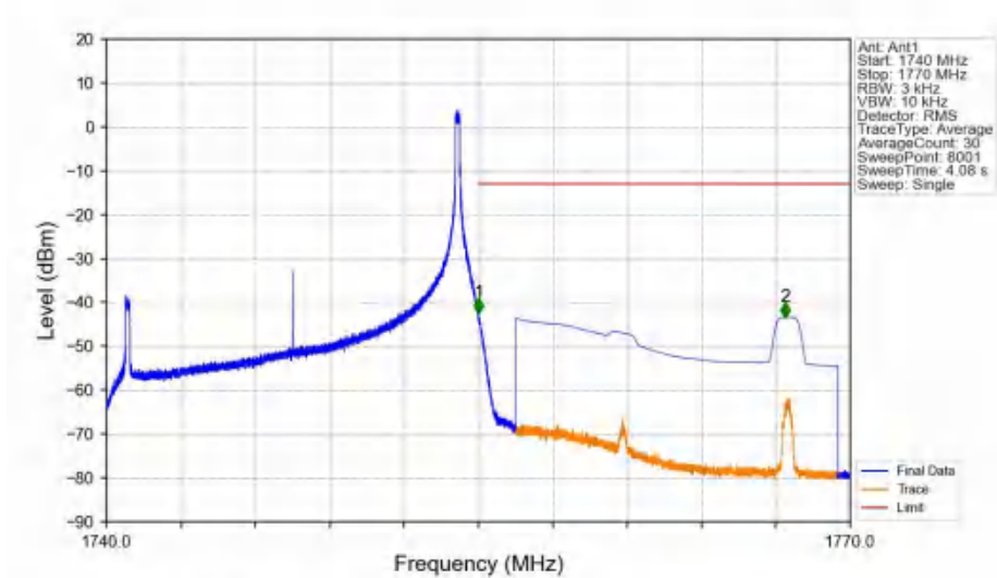
Band4_15MHz_QPSK_HCH_1747.5MHz_RB_1_74_NTNV
