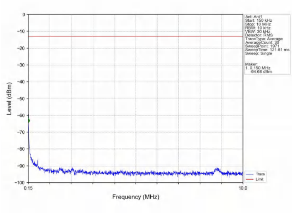
Band4_10MHz_QPSK_HCH_1750MHz_RB_1_0_NTNV
