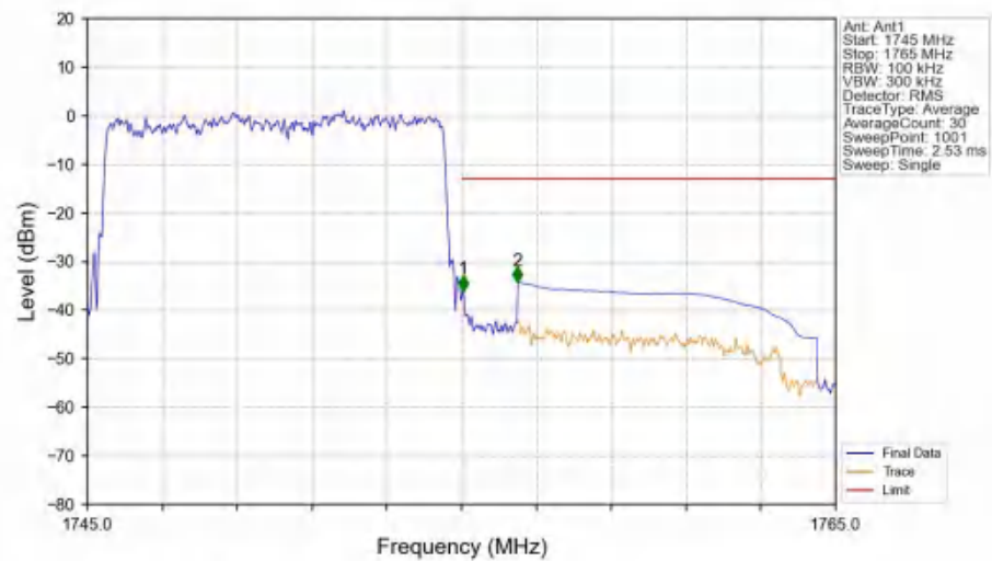
Band4_10MHz_QPSK_HCH_1750MHz_RB_50_0_NTNV
