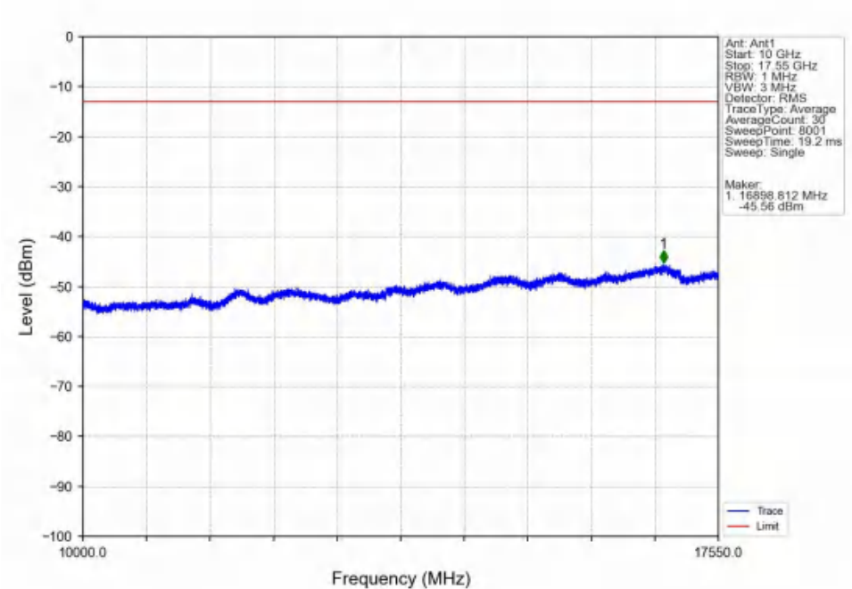
Band4_15MHz_QPSK_LCH_1717.5MHz_RB_1_0_NTNV
