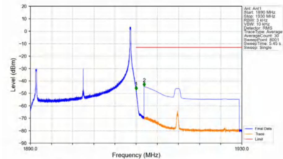
Band2_20MHz_QPSK_HCH_1900MHz_RB_1_99_NTNV
