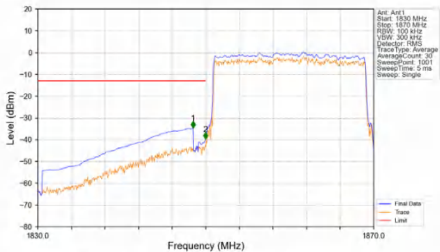
Band2_20MHz_16QAM_LCH_1860MHz_RB_100_0_NTNV
