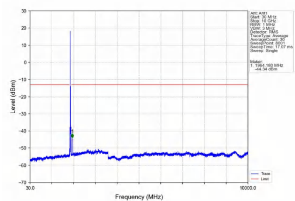
Band2_20MHz_QPSK_MCH_1880MHz_RB_1_0_NTNV
