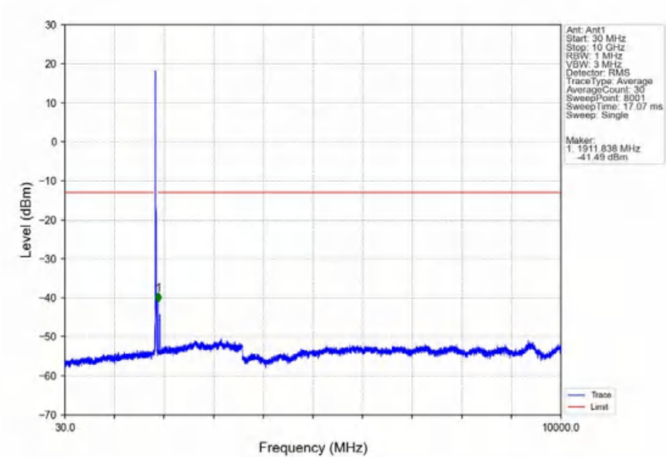
Band2_20MHz_QPSK_LCH_1860MHz_RB_1_0_NTNV
