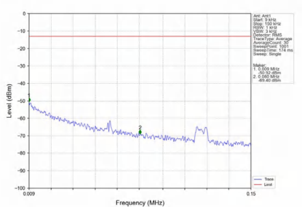
Band2_20MHz_QPSK_MCH_1880MHz_RB_1_0_NTNV
