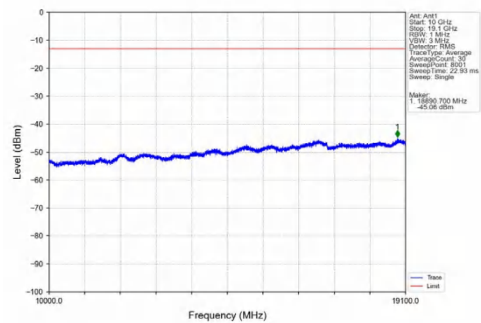
Band2_20MHz_QPSK_HCH_1900MHz_RB_1_99_NTNV
