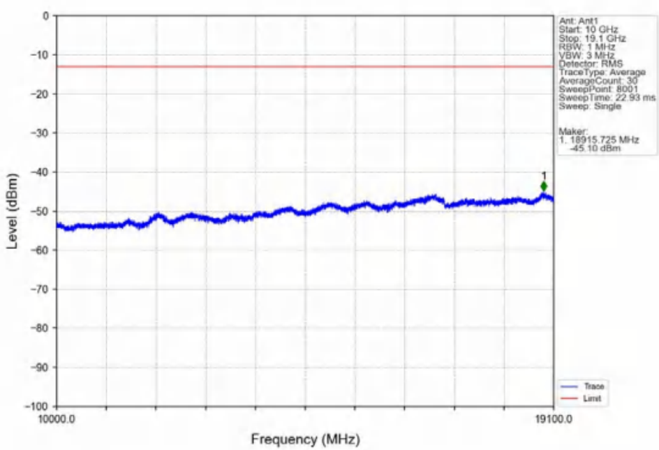
Band2_20MHz_16QAM_HCH_1900MHz_RB_1_0_NTNV
