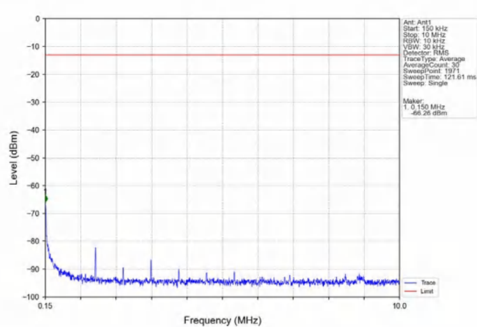
Band2_20MHz_16QAM_MCH_1880MHz_RB_1_0_NTNV
