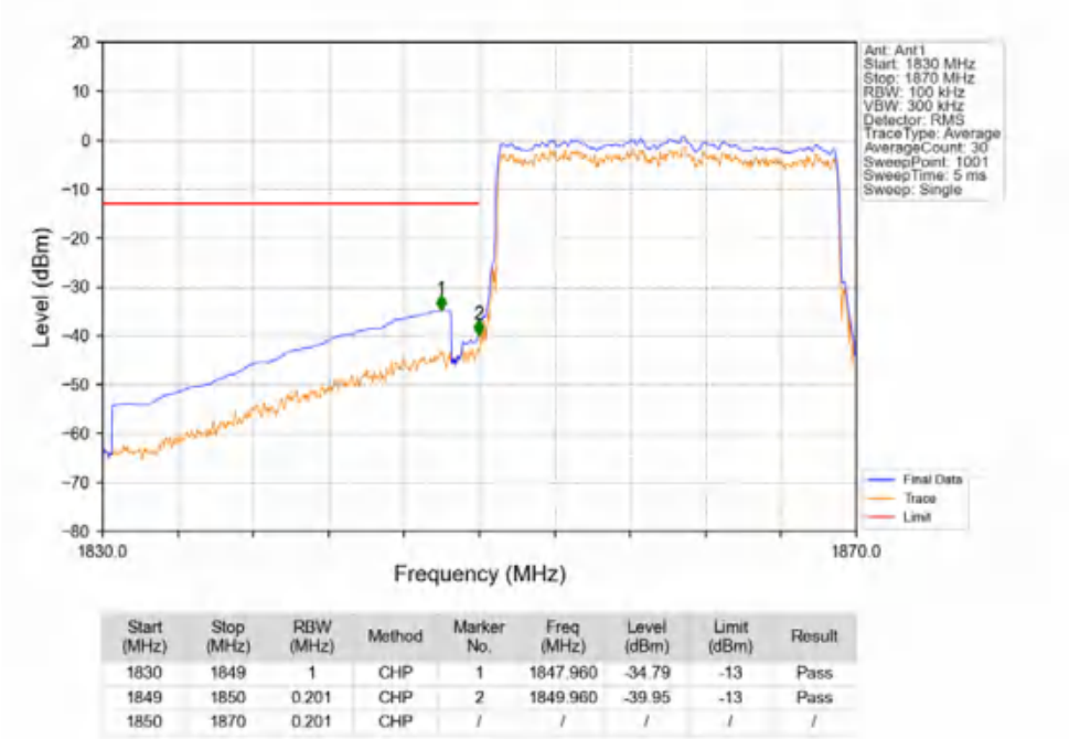
Band2_20MHz_QPSK_LCH_1860MHz_RB_100_0_NTNV
