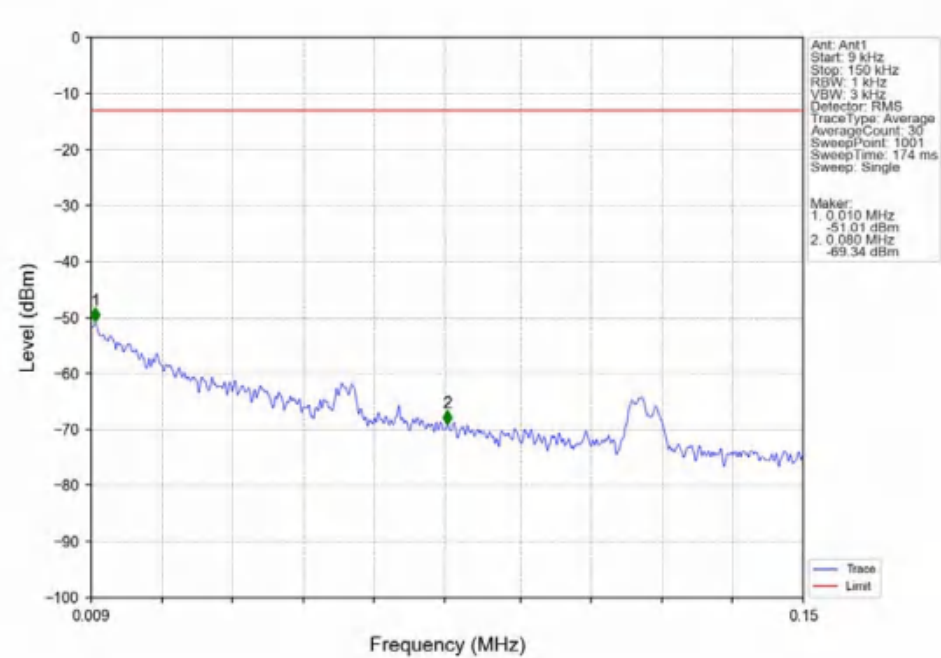
Band2_20MHz_16QAM_MCH_1880MHz_RB_1_0_NTNV
