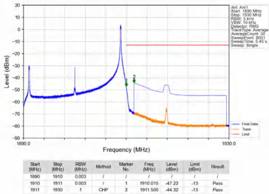
Band2_20MHz_16QAM_HCH_1900MHz_RB_100_0_NTNV
