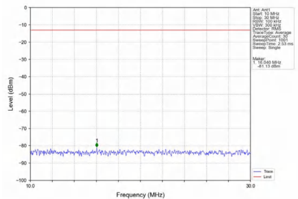
Band2_3MHz_16QAM_MCH_1880MHz_RB_1_0_NTNV
