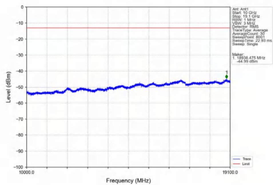
Band2_1.4MHz_QPSK_HCH_1909.3MHz_RB_1_5_NTNV
