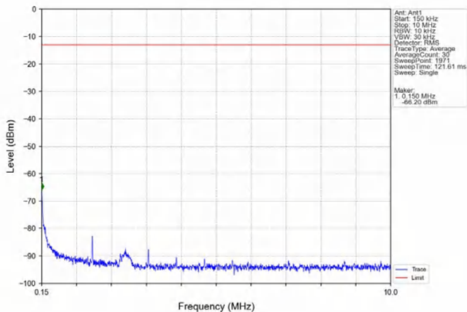
Band2_3MHz_16QAM_MCH_1880MHz_RB_1_0_NTNV
