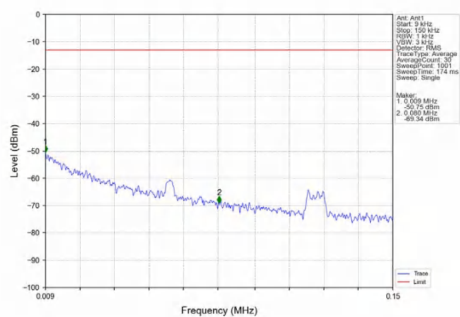
Band2_3MHz_QPSK_MCH_1880MHz_RB_1_0_NTNV
