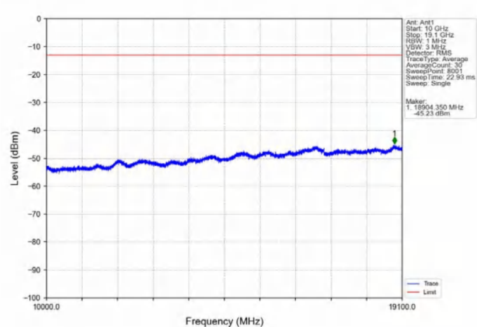
Band2_15MHz_QPSK_MCH_1880MHz_RB_1_0_NTNV
