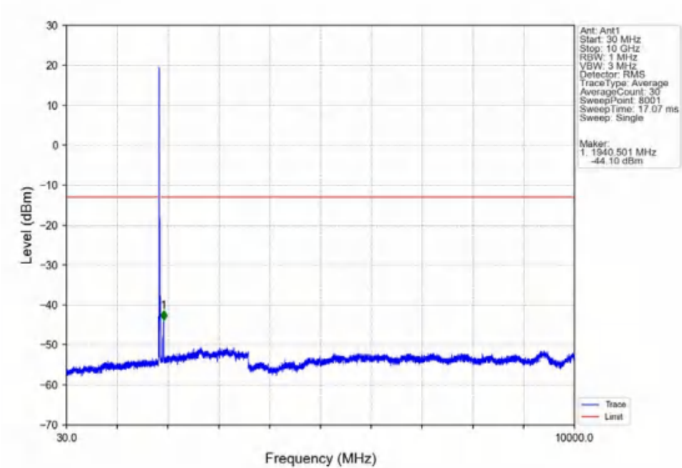
Band2_15MHz_QPSK_LCH_1857.5MHz_RB_1_0_NTNV
