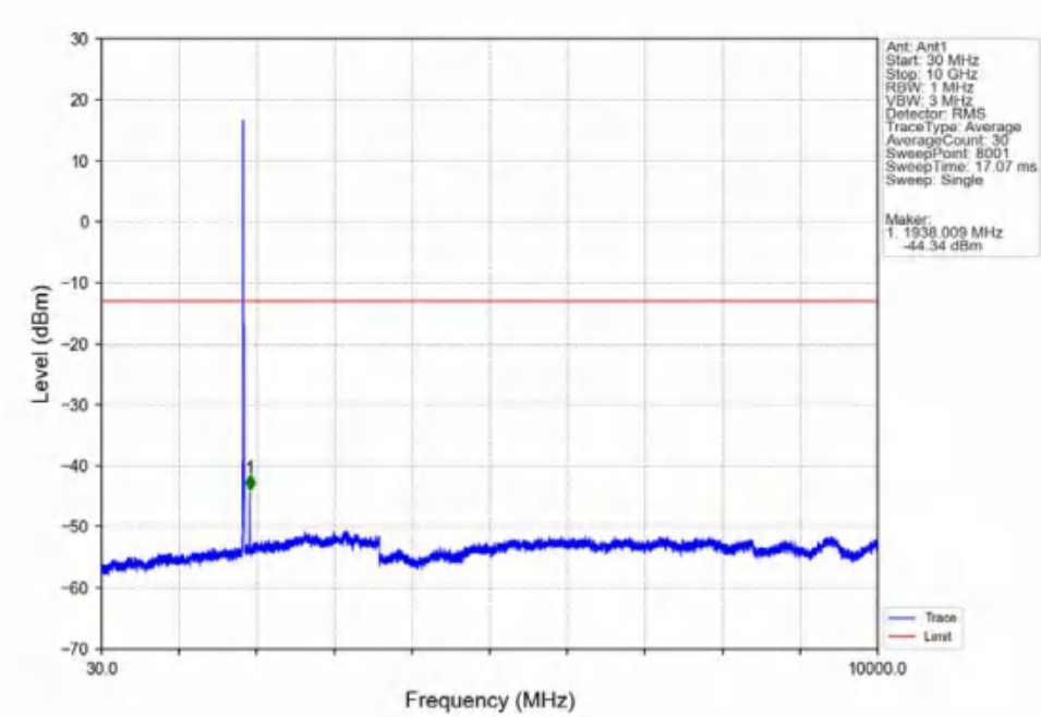
Band2_10MHz_QPSK_LCH_1855MHz_RB_1_0_NTNV
