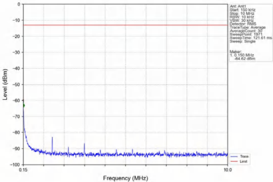
Band2_15MHz_QPSK_LCH_1857.5MHz_RB_1_0_NTNV
