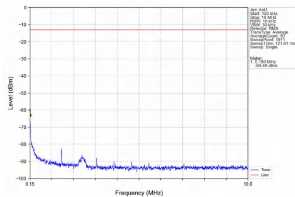
Band2_3MHz_QPSK_LCH_1851.5MHz_RB_1_0_NTNV
