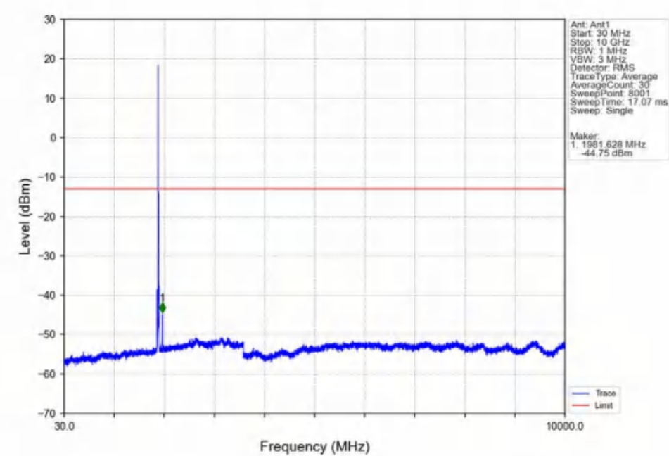
Band2_10MHz_QPSK_HCH_1905MHz_RB_1_0_NTNV
