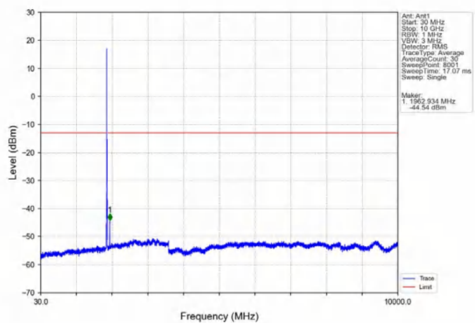
Band2_10MHz_QPSK_MCH_1880MHz_RB_1_0_NTNV
