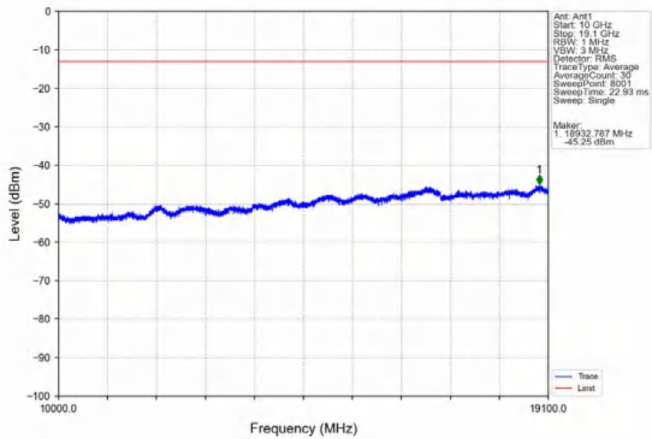
Band2_10MHz_QPSK_HCH_1905MHz_RB_1_49_NTNV
