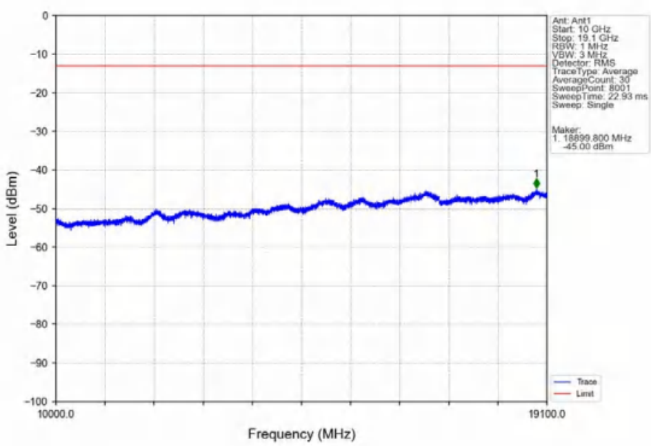
Band2_3MHz_QPSK_LCH_1851.5MHz_RB_1_0_NTNV
