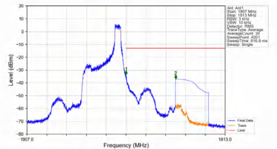
Band2_1.4MHz_QPSK_HCH_1909.3MHz_RB_1_5_NTNV
