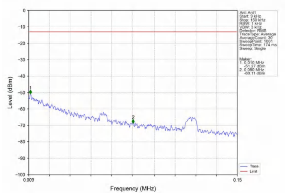
Band2_5MHz_QPSK_MCH_1880MHz_RB_1_0_NTNV
