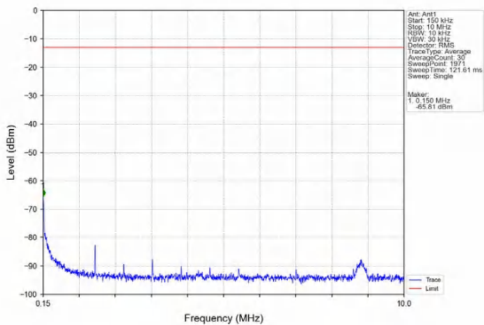
Band2_10MHz_16QAM_LCH_1855MHz_RB_1_0_NTNV
