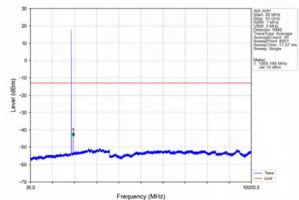
Band2_3MHz_16QAM_MCH_1880MHz_RB_1_0_NTNV
