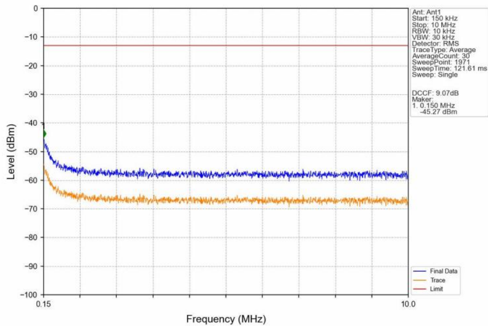
GSM850_GSM_HCH_848.8MHz_GSM_NTNV
