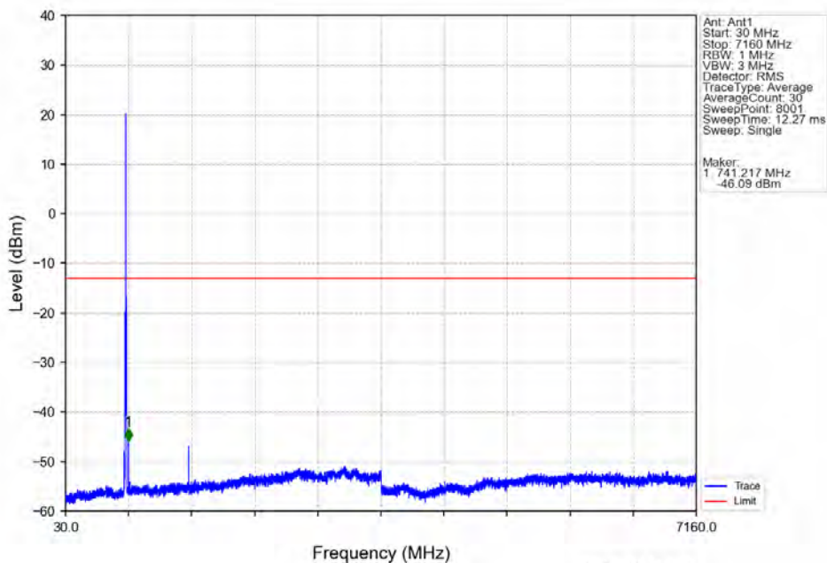
Band12 5MHz QPSK HCH 713.5MHz RB 1 24 NTNV
