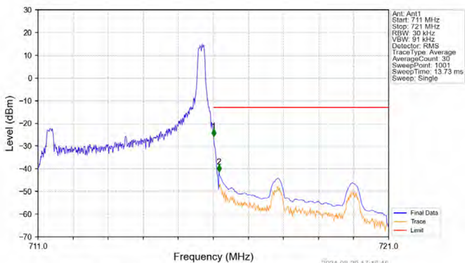
Band12 5MHz QPSK HCH 713.5MHz RB 1 24 NTNV
