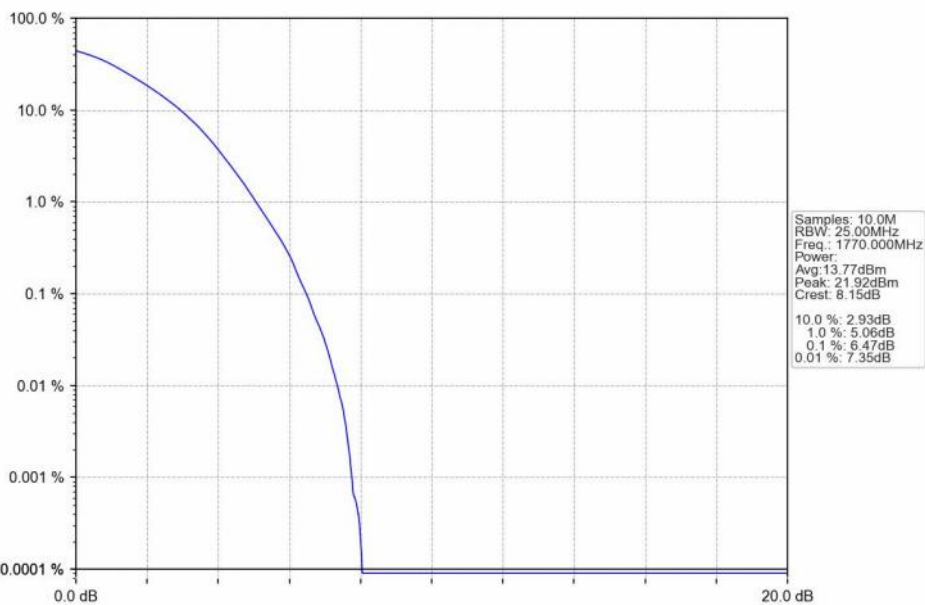
n66_30kHz_SISO_NTNV_20MHz_DFT-s-OFDM_256_QAM_1770MHz_Outer_Full_Ant1
