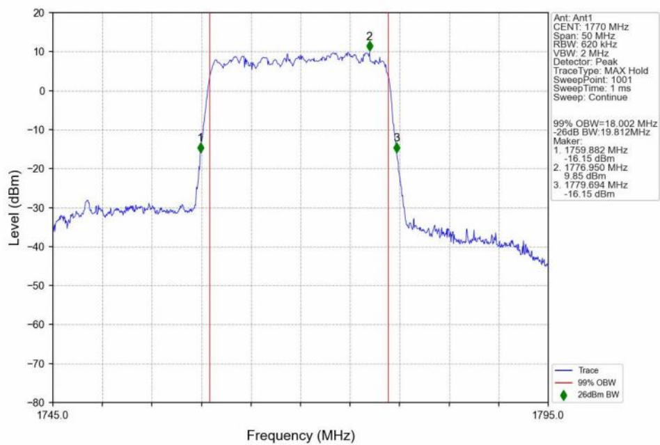
n66_30kHz_SISO_NTNV_20MHz_DFT-s-OFDM_256_QAM_1770MHz_Outer_Full_Ant1
