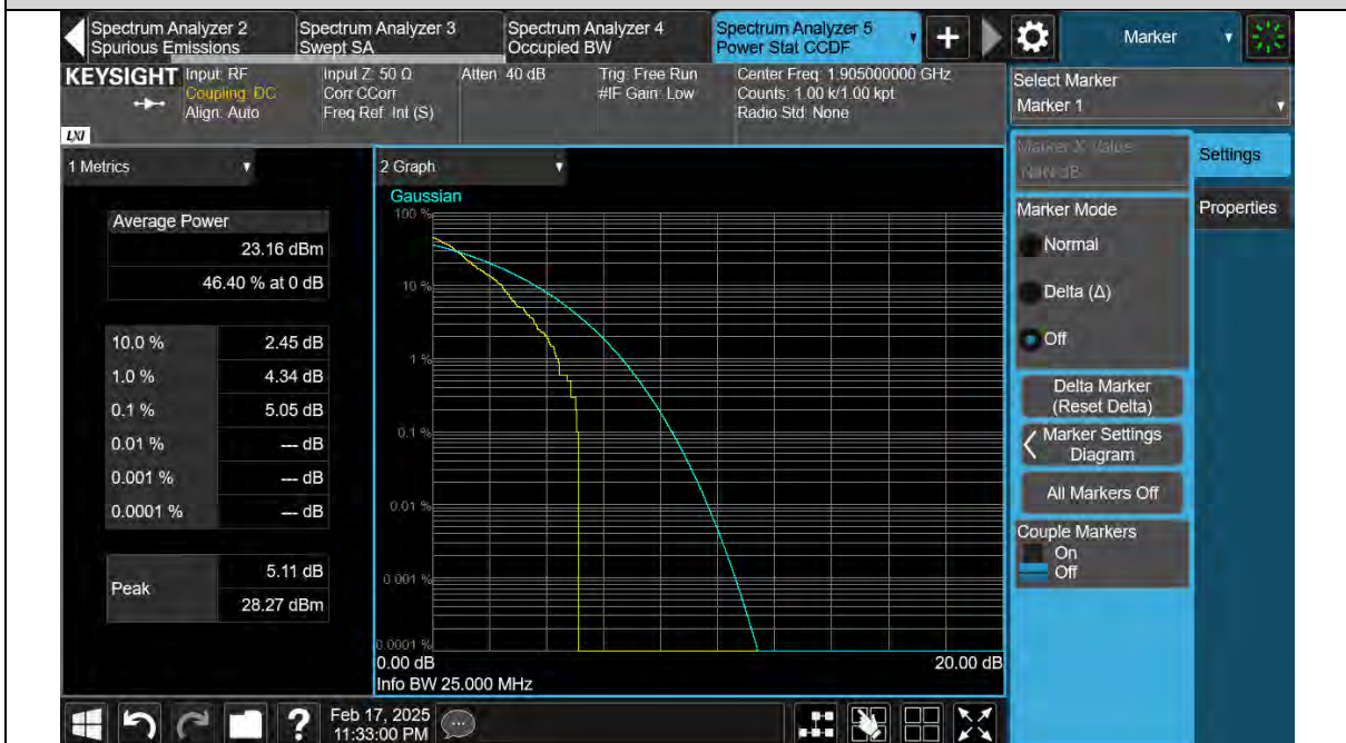
Band25-20MHz-QPSK-26590-100RB#0
