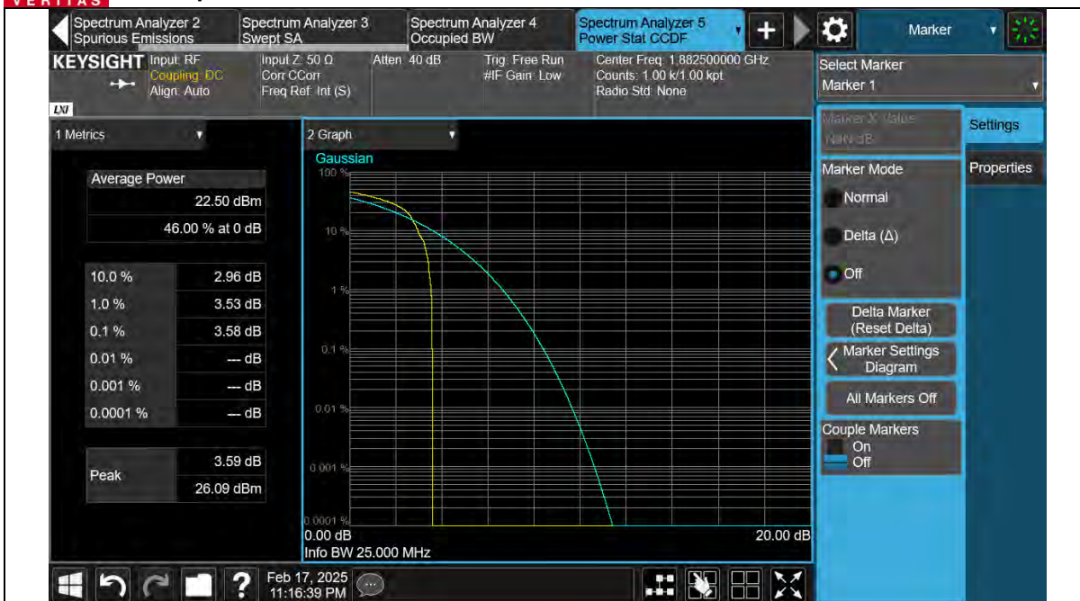
Band25-20MHz-QPSK-26365-1RB#0
