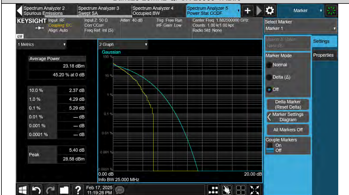
Band25-20MHz-QPSK-26365-100RB#0
