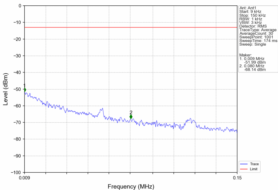
Band4 HSUPA LCH 1712.4MHz Subtest 1 NTNV
