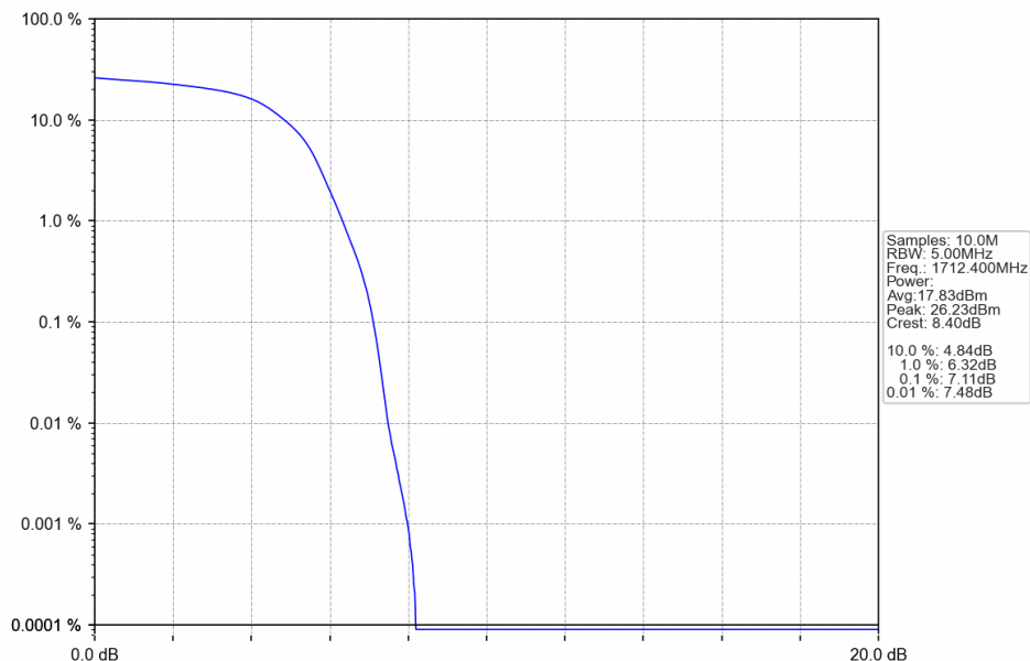
Band4 HSUPA LCH 1712.4MHz Subtest 1 NTV
