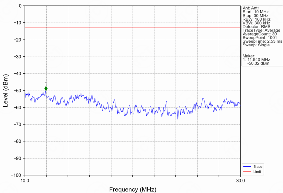
Band4 1.4MHz QPSK LCH 1710.7MHz RB 1 0 NTNV
