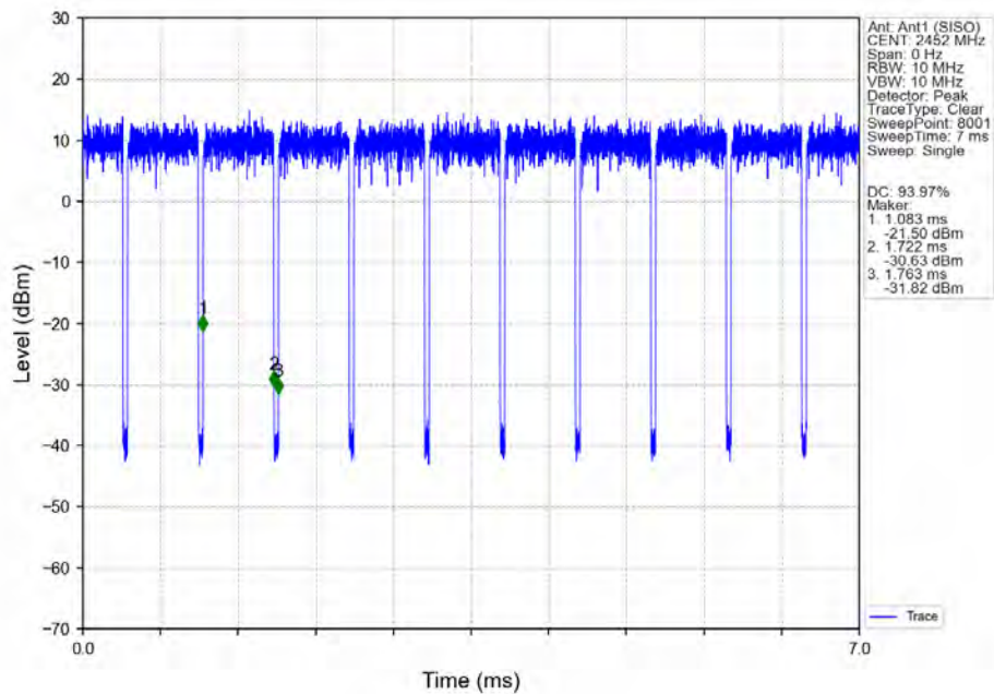
802.11n(HT40)_HCH_2452MHz_Ant1 (SISO)_NTNV
