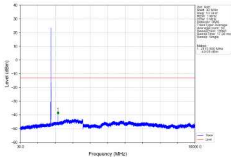
Band66 10MHz QPSK HCH 1775MHz RB 1 0 NTNV
