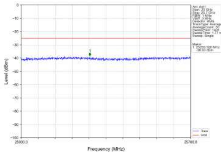
Band7_5MHz_QPSK_MCH_2535MHz_RB_1_0_NTNV
