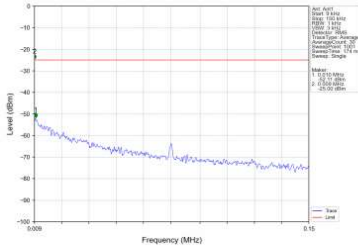
Band7_20MHz_16QAM_MCH_2535MHz_RB_1_0_NTNV
