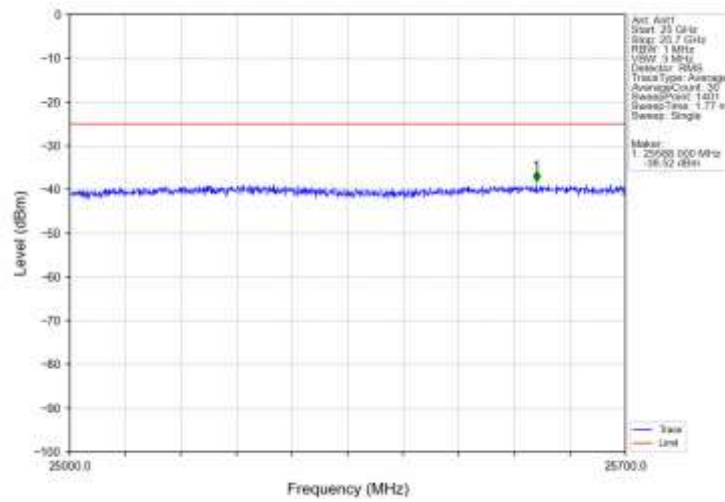
Band7_10MHz_QPSK_MCH_2535MHz_RB_1_0_NTNV
