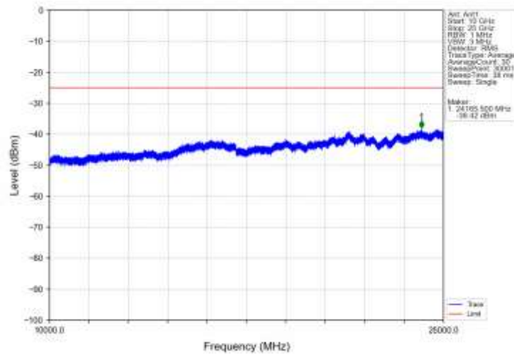
Band7_10MHz_QPSK_MCH_2535MHz_RB_1_0_NTNV
