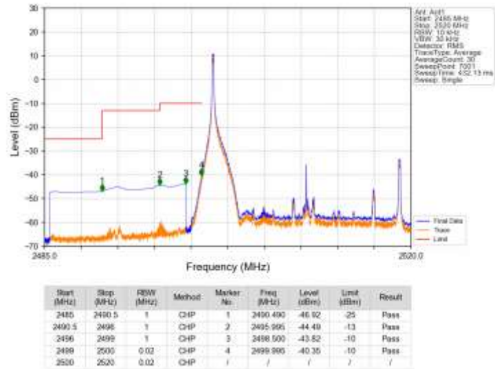
Band7_20MHz_QPSK_LCH_2510MHz_RB_1_0_NTNV
