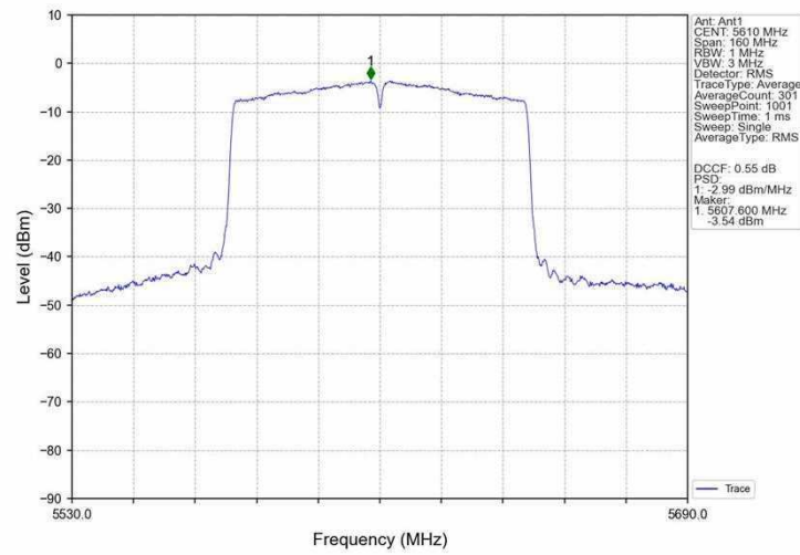
802.11ac(VHT80)_HCH_5610MHz_Ant1_NTNV
