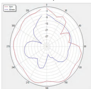
H Theta=90 freq=2020MHz
