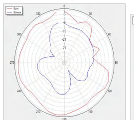
H Theta=90 freq=1960MHz
