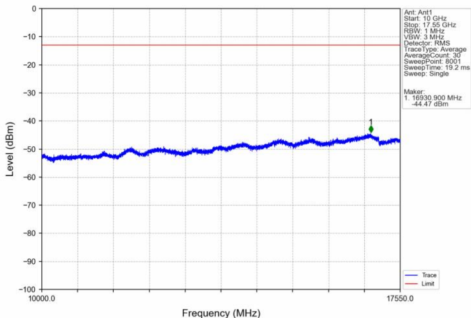
Band4_10MHz_QPSK_HCH_1750MHz_RB_1_49_NTNV
