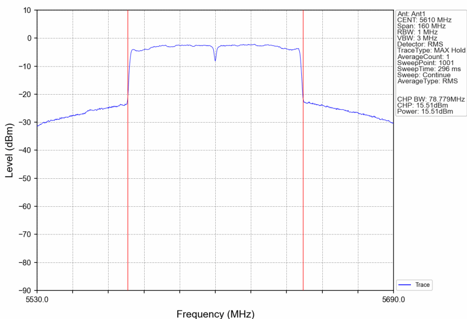
802.11ac(VHT80) HCH 5610MHz Ant1 NTN
