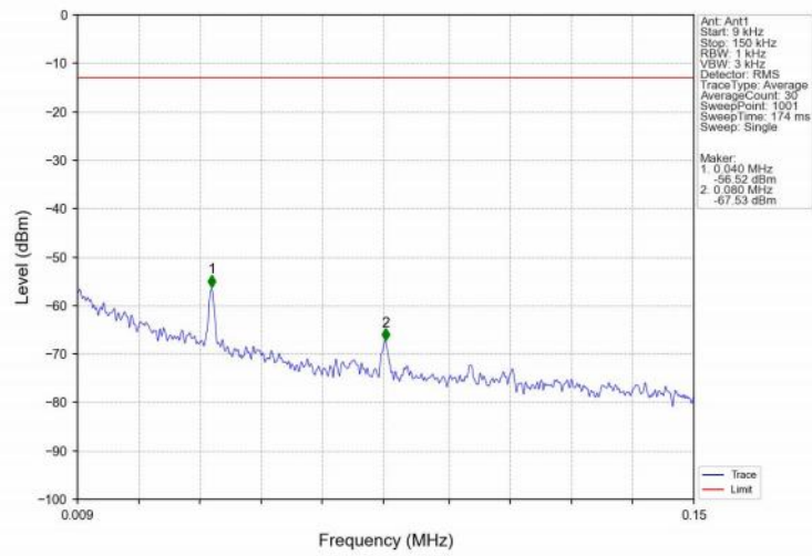
Band71_5MHz_QPSK_HCH_695.5MHz_RB_1_0_NTNV
