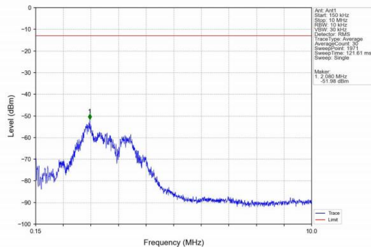
Band71_20MHz_QPSK_HCH_688MHz_RB_1_0_NTNV
