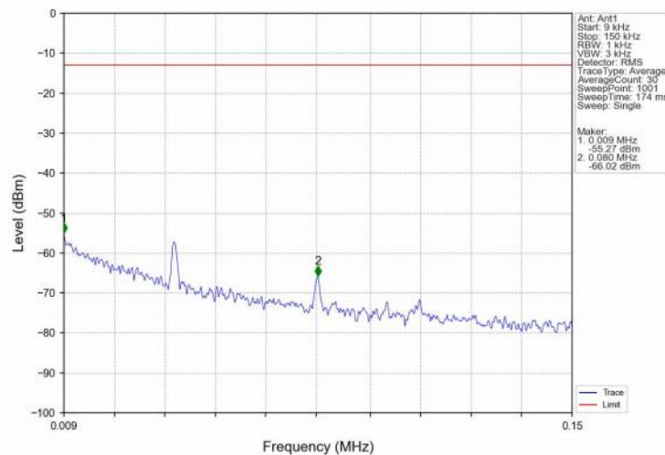
Band71_20MHz_QPSK_LCH_673MHz_RB_1_0_NTNV
