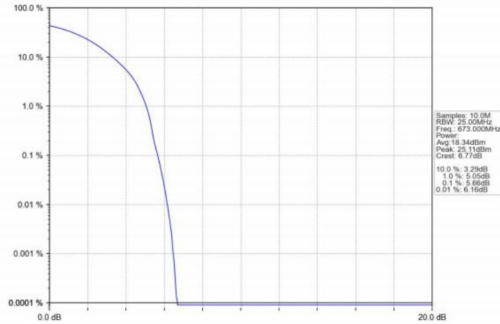
Band71_20MHz_QPSK_LCH_673MHz_RB_100_0_NTNV
