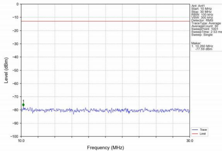
Band71_5MHz_16QAM_LCH_665.5MHz_RB_1_0_NTNV
