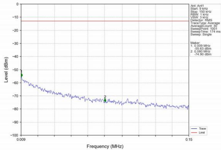
Band71_20MHz_16QAM_HCH_688MHz_RB_1_0_NTNV
