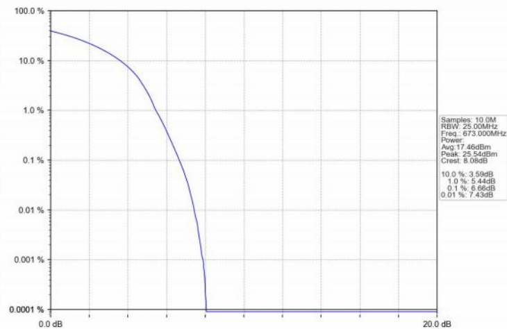
Band71_20MHz_16QAM_LCH_673MHz_RB_100_0_NTNV
