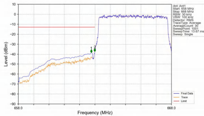
Band71_5MHz_QPSK_LCH_665.5MHz_RB_25_0_NTNV
