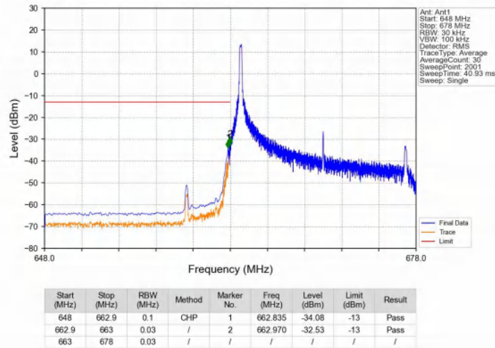
Band71_15MHz_QPSK_LCH_670.5MHz_RB_1_0_NTNV
