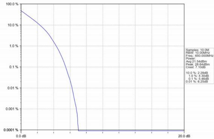
Band71_10MHz_QPSK_HCH_693MHz_RB_50_0_NTNV
