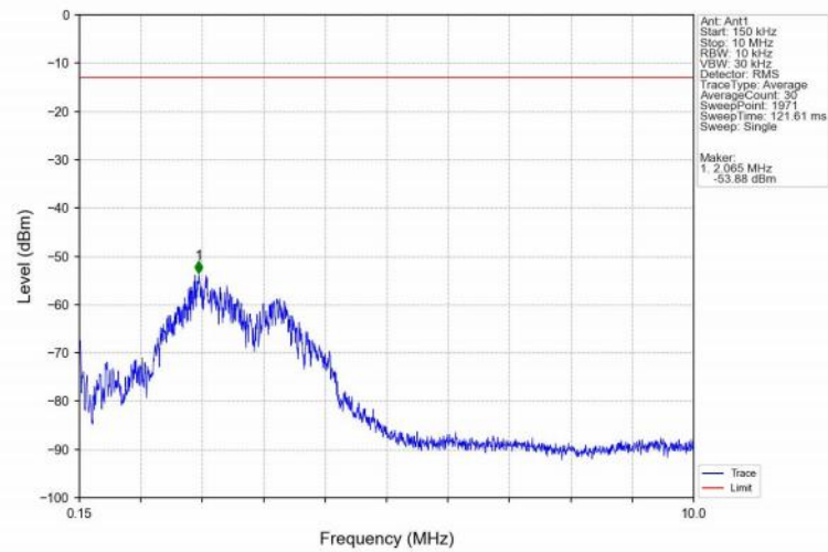
Band71_10MHz_QPSK_LCH_668MHz_RB_1_0_NTNV
