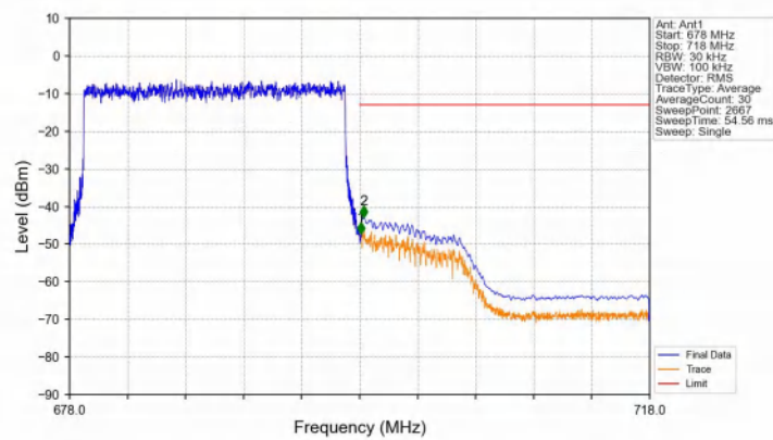
Band71_20MHz_16QAM_HCH_688MHz_RB_100_0 NTNv
