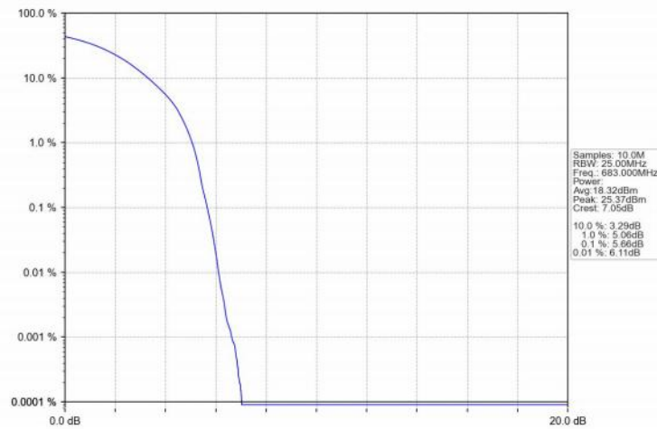
Band71_20MHz_QPSK_MCH_683MHz_RB_100_0_NTNV
