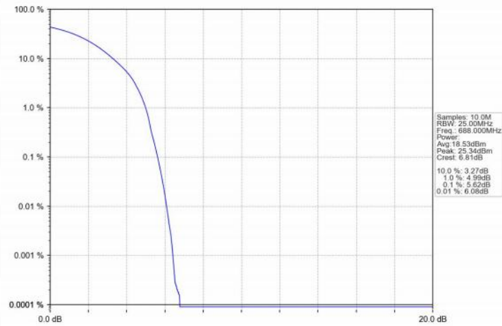
Band71_20MHz_QPSK_HCH_688MHz_RB_100_0_NTNV
