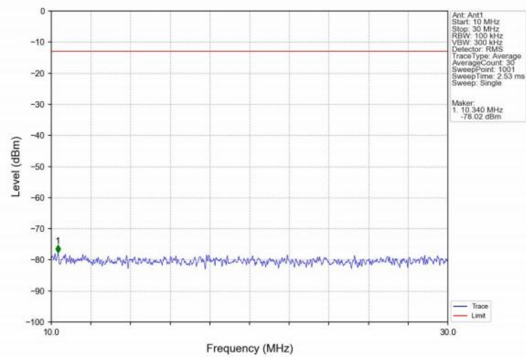
Band71_20MHz_QPSK_HCH_688MHz_RB_1_0_NTNV
