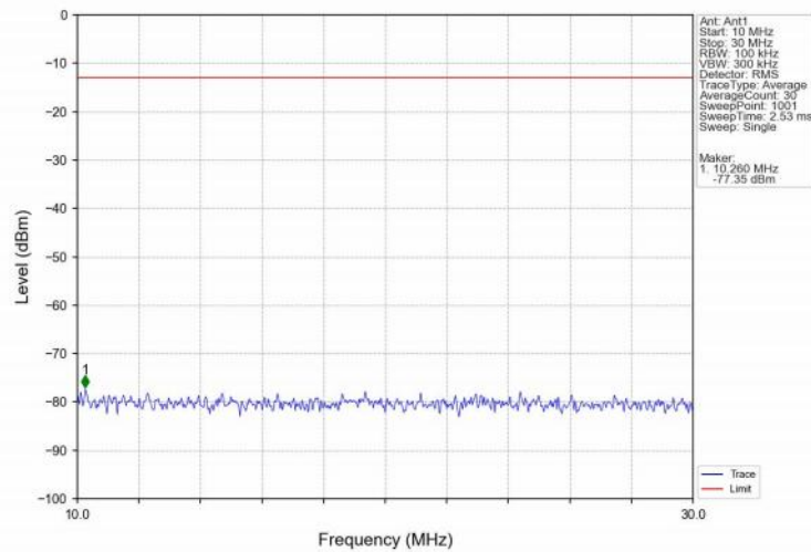
Band71_20MHz_16QAM_LCH_673MHz_RB_1_0_NTNV
