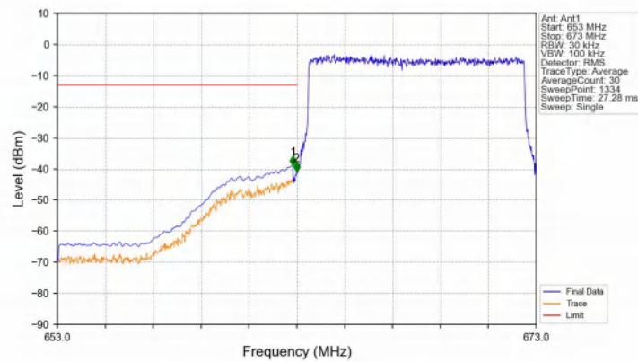
Band71_10MHz_QPSK_LCH_668MHz_RB_50_0_NTNV
