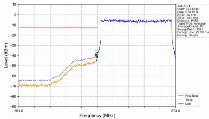
Band71_10MHz_16QAM_LCH_668MHz_RB_50_0_NTNV
