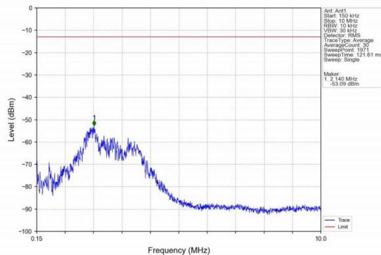
Band71_10MHz_QPSK_HCH_693MHz_RB_1_0_NTNV
