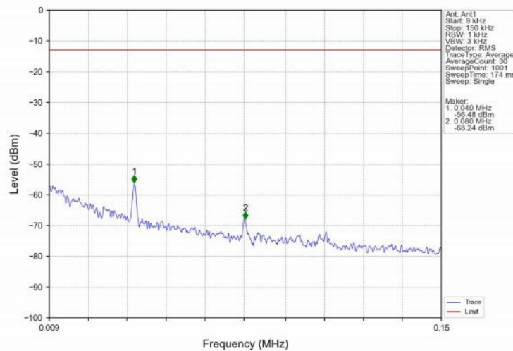
Band71_5MHz_QPSK_LCH_665.5MHz_RB_1_0_NTNV
