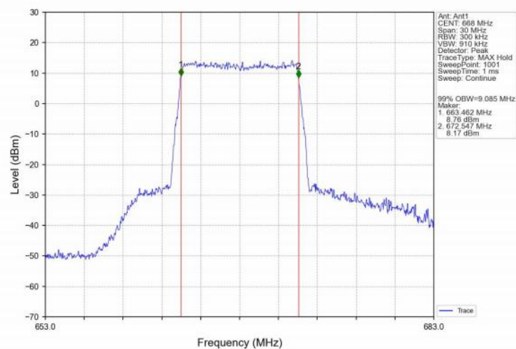
Band71_10MHz_16QAM_LCH_668MHz_RB_50_0_NTNV
