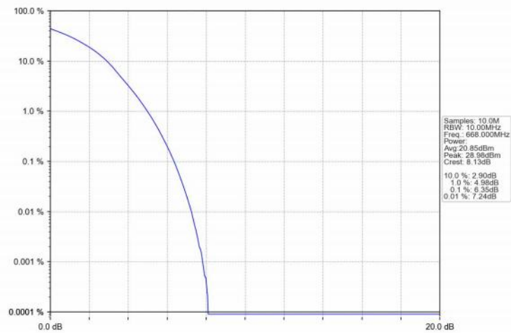
Band71_10MHz_16QAM_LCH_668MHz_RB_50_0_NTNV
