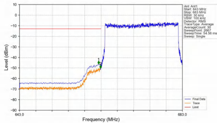
Band71_20MHz_16QAM_LCH_673MHz_RB_100_0_NTNV
