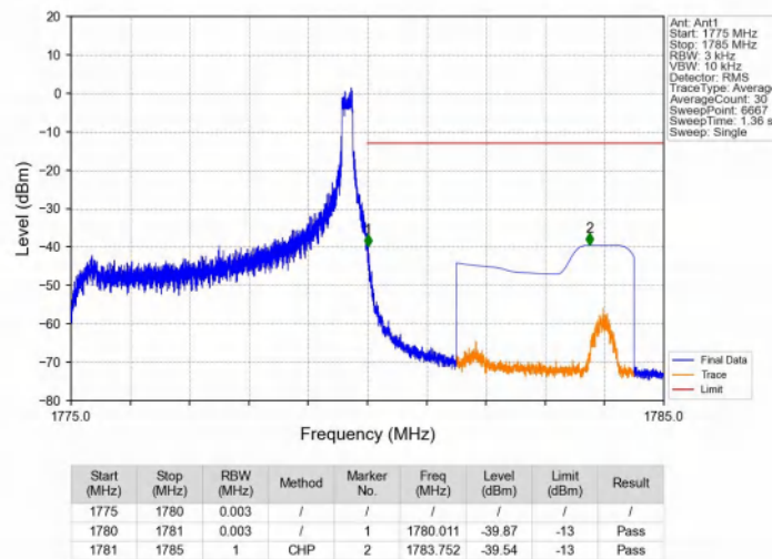
Band66_5MHz_QPSK_HCH_1777.5MHz_RB_1_24_NTNV
