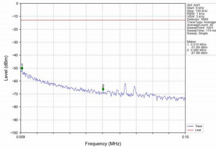
Band66_20MHz_QPSK_LCH_1720MHz_RB_1_0_NTNV
