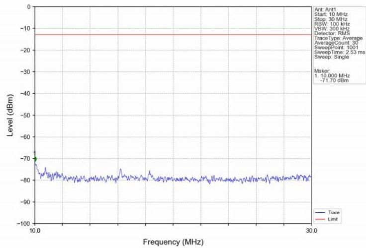
Band25_20MHz_QPSK_HCH_1905MHz_RB_1_0_NTNV
