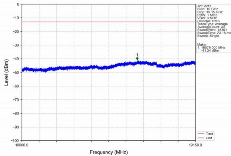
Band25_10MHz_QPSK_HCH_1910MHz_RB_1_49_NTNV
