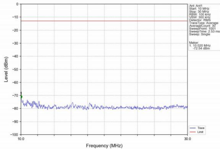
Band25_10MHz_QPSK_LCH_1855MHz_RB_1_0_NTNV
