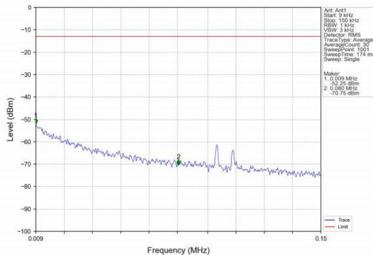
Band25_10MHz_QPSK_LCH_1855MHz_RB_1_0_NTNV
