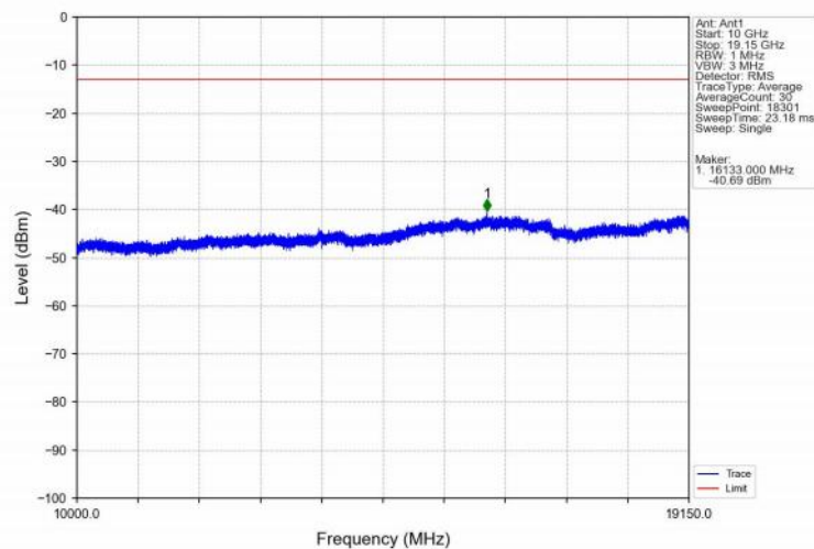
Band25_10MHz_QPSK_LCH_1855MHz_RB_1_0_NTNV
