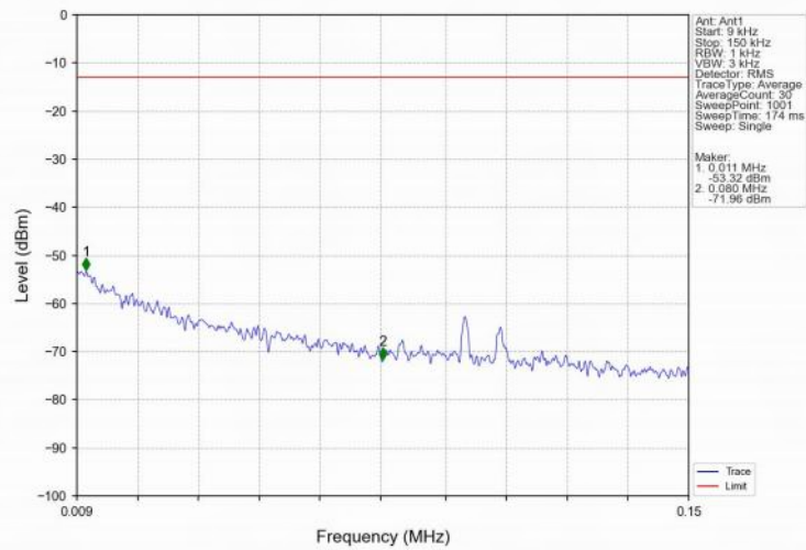
Band25_20MHz_QPSK_HCH_1905MHz_RB_1_0_NTNV
