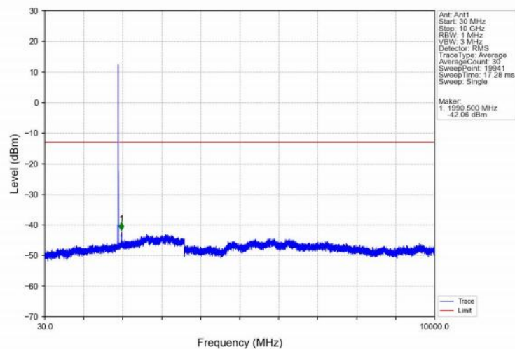
Band25_10MHz_QPSK_HCH_1910MHz_RB_1_0_NTNV
