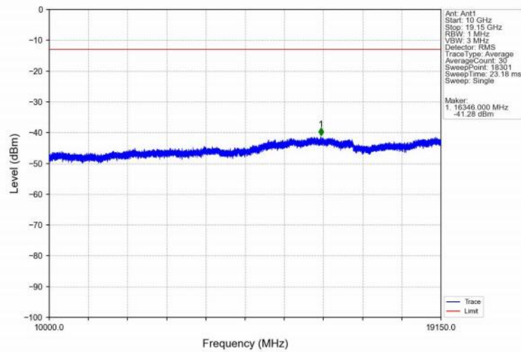
Band25_20MHz_QPSK_HCH_1905MHz_RB_1_99_NTNV
