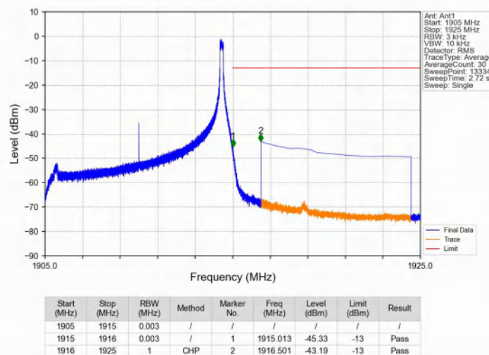
Band25_10MHz_QPSK_HCH_1910MHz_RB_1_49_NTNV
