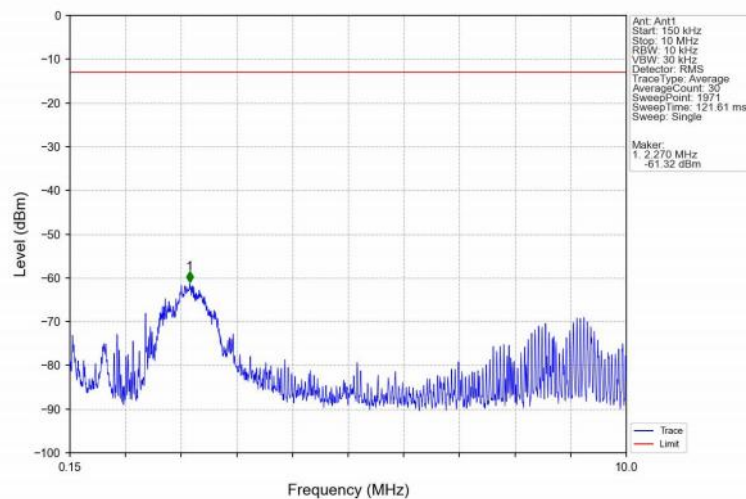
Band25_10MHz_QPSK_HCH_1910MHz_RB_1_0_NTNV
