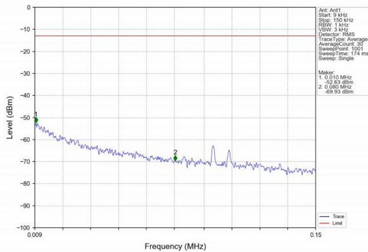
Band25_20MHz_QPSK_LCH_1860MHz_RB_1_0_NTNV
