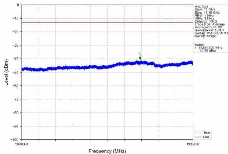
Band25_20MHz_QPSK_LCH_1860MHz_RB_1_0_NTNV
