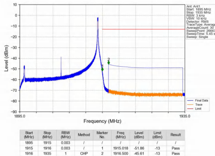
Band25_20MHz_QPSK_HCH_1905MHz_RB_1_99_NTNV
