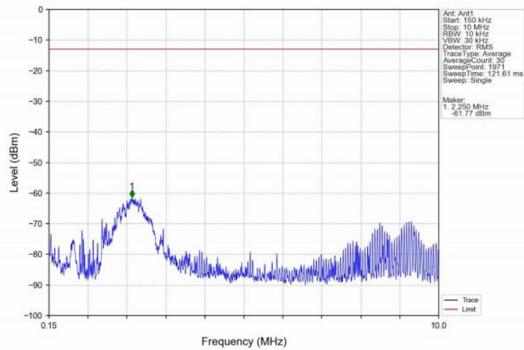
Band25_20MHz_QPSK_LCH_1860MHz_RB_1_0_NTNV
