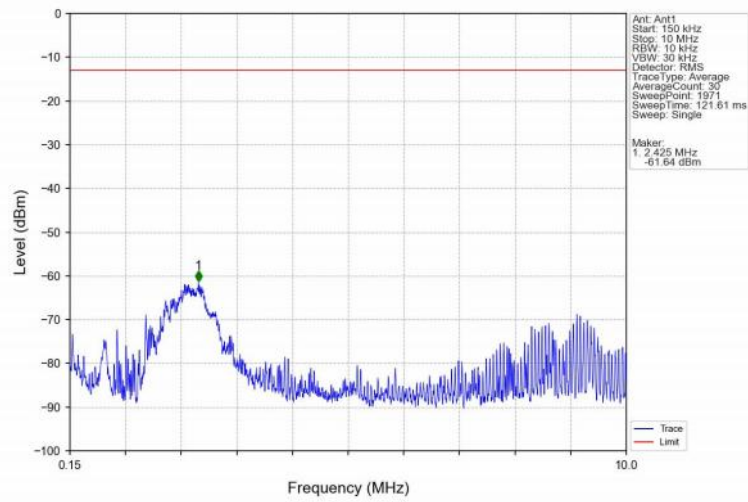
Band25_10MHz_QPSK_LCH_1855MHz_RB_1_0_NTNV
