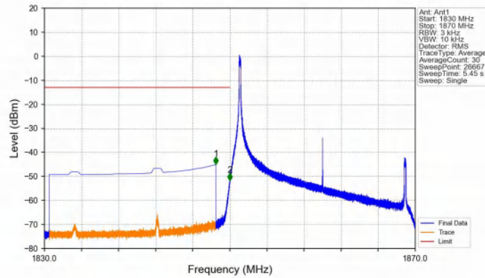
Band25_20MHz_QPSK_LCH_1860MHz_RB_1_0_NTNV
