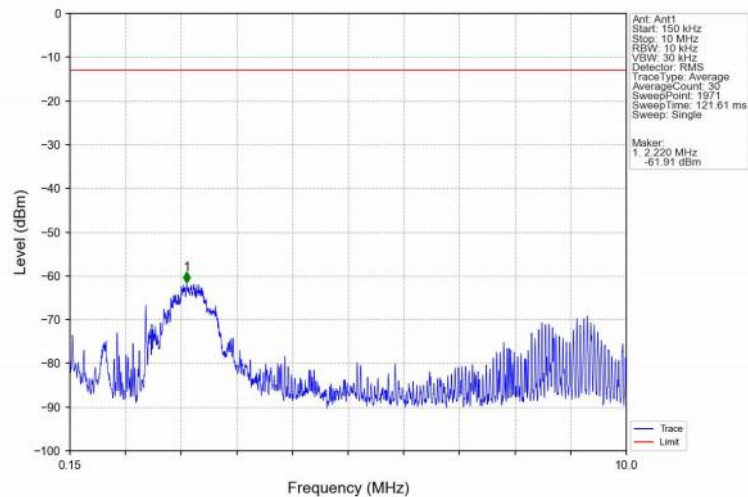
Band25_20MHz_QPSK_HCH_1905MHz_RB_1_0_NTNV
