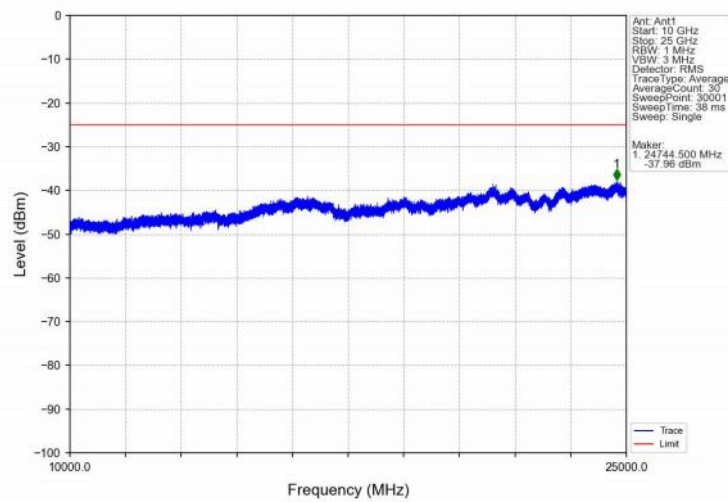
Band7_5MHz_QPSK_HCH_2567.5MHz_RB_1_0_NTNV
