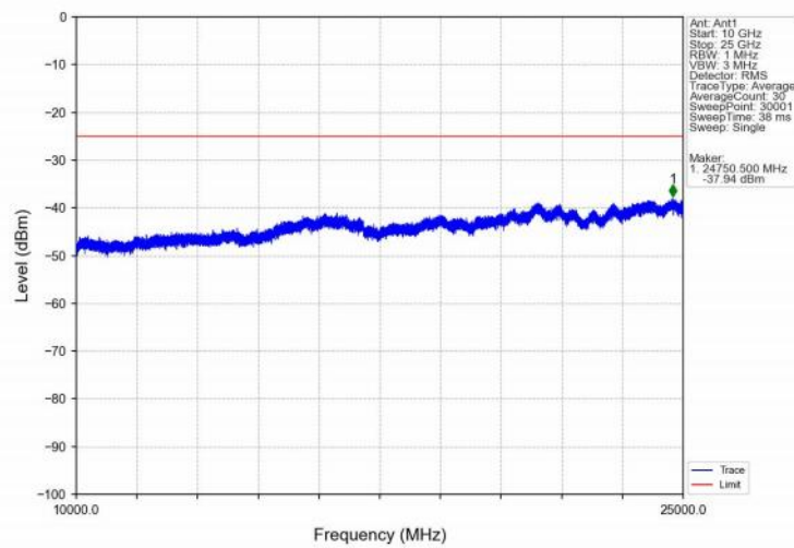
Band7_10MHz_QPSK_MCH_2535MHz_RB_1_0_NTNV
