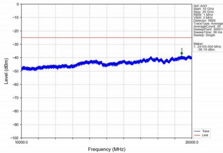
Band7_10MHz_QPSK_HCH_2565MHz_RB_1_0_NTNV
