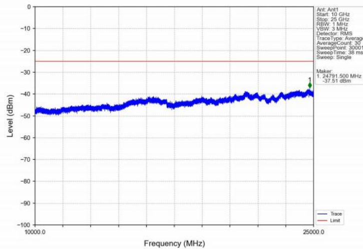
Band7_5MHz_QPSK_LCH_2502.5MHz_RB_1_0_NTNV
